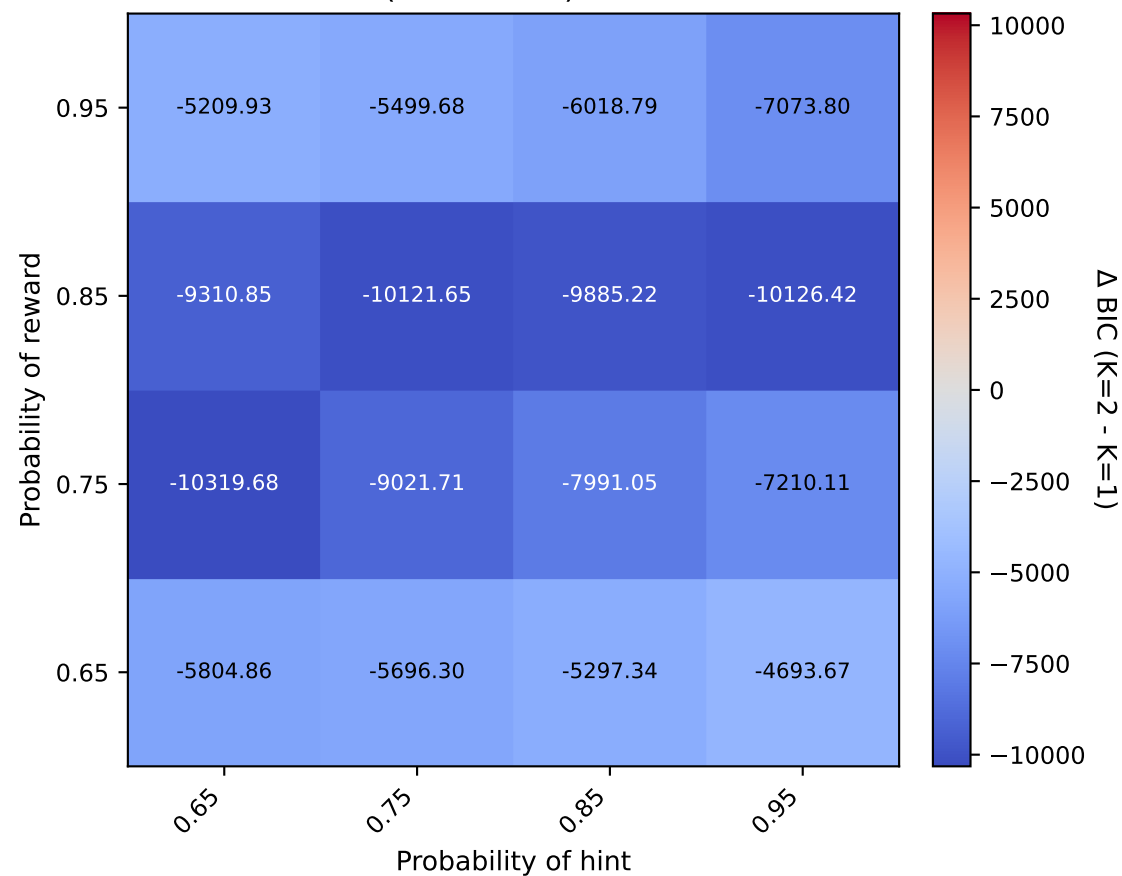
\Delta BIC (K=2 - K=1) — Case C
