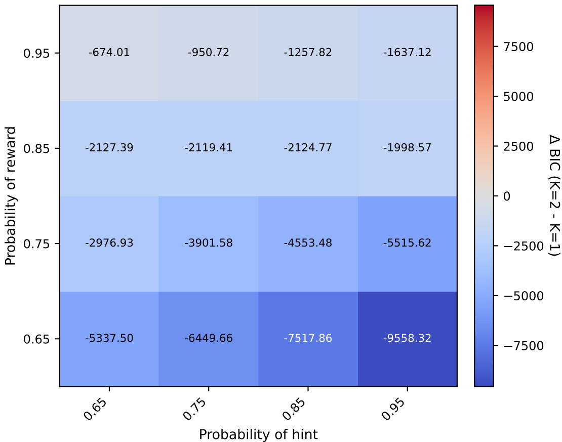
\Delta BIC (K=2 - K=1) — Case A
