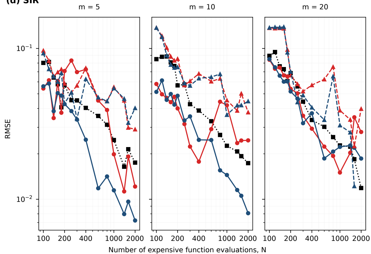
(d) SIR
