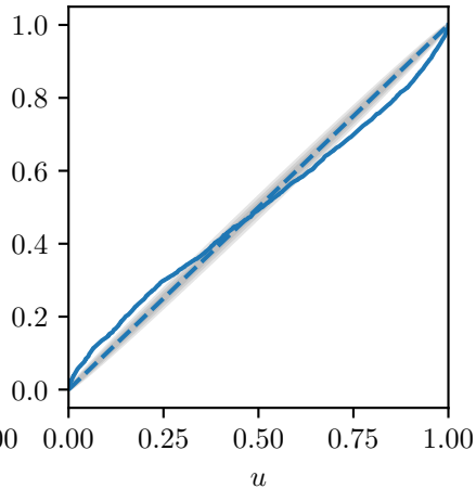
CDF P(u)
