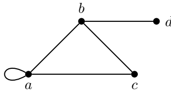
Figura 2.2: Grafo con lazo en el vértice a.
