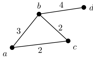
Figura 2.4: Grafo ponderado.
