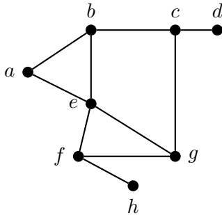
Figura 2.9: Grafo G
