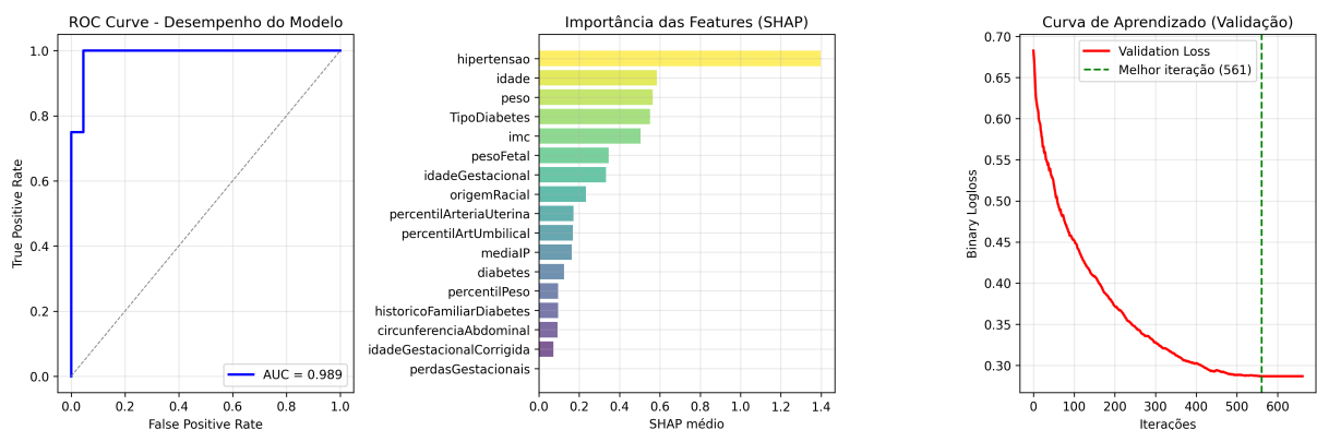
Figura 4 – Métricas de avaliação do modelo LightGBM: curva ROC, importância das variáveis e curva de aprendizado.
