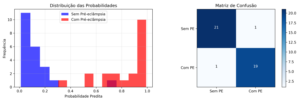
Figura 5 – Distribuição de probabilidades previstas e matriz de confusão do modelo LightGBM.
