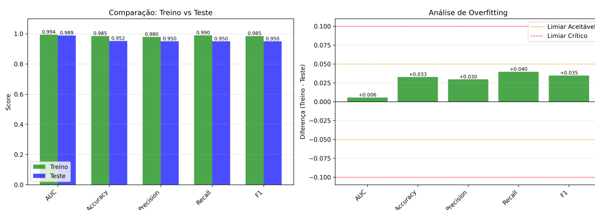
Figura 6 – Análise de sobreajuste: comparação entre métricas de treino e teste do modelo LightGBM.
