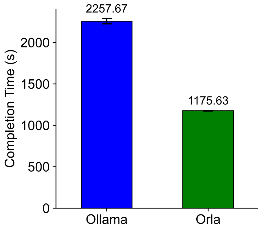
(b) Edge Serving
