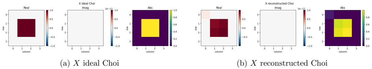
Figure 3: X gate의 이상적인 Choi 행렬과 재구성된 Choi 행렬 비교. 두 그림의 큰 구조는 비슷하지만 재구성된 행렬에서는 ideal pattern에서 벗어난 작은 성분들이 나타난다. 이는 gate가 완전히 틀렸다는 뜻이 아니라, 이상적인 unitary 과정에 잡음 성분이 섞였다는 뜻으로 해석된다.
