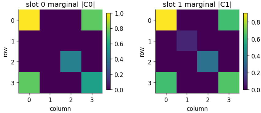
Figure 10: Two-use comb의 각 slot marginal Choi 행렬. 각 marginal만 보면 정상적인 single-step channel처럼 보이지만, marginal들의 곱만으로 전체 comb를 재구성할 수 없었다. 따라서 memory effect는 개별 시점의 채널이 아니라 시점 사이의 correlation에서 나타난다.
