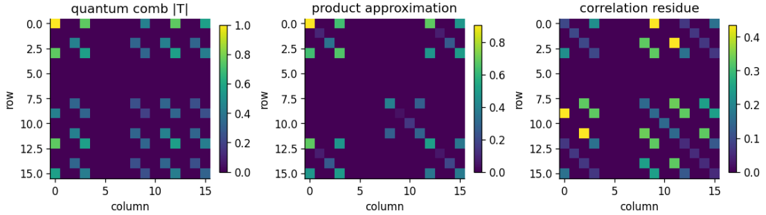
Fig 9. Two-use collision model의 comb(좌), memoryless product(중), 그리고 둘의 차이(우). 차이가 0이 아니면 시점 간 correlation이 존재함을 뜻하며, 독립적 두 channel의 연속으로 설명되지 않는다고 생각된다
