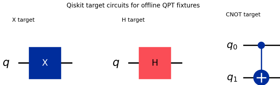
Fig 2. Offline QPT fixture의 target circuits. X, H는 1큐비트, CNOT은 2큐비트이다. Noise는 target gate 뒤의 Choi-level channel로 적용했다
