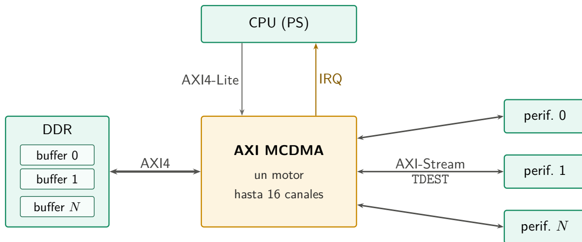
Figura 2.9: Transferencia multicanal con AXI MCDMA.
