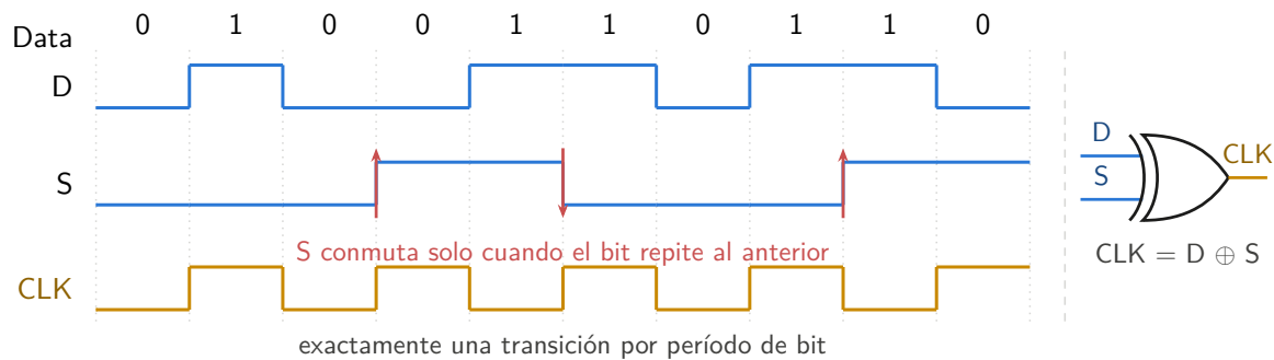
Figura 2.4: Codificación Data-Strobe y recuperación del reloj.
