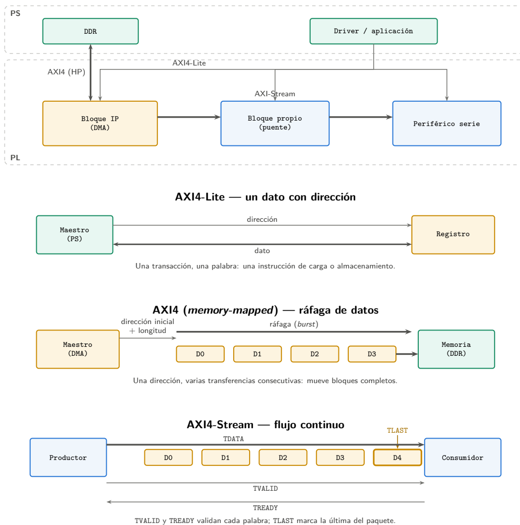
Figura 2.3: Perfiles del bus AXI4 y su uso entre el PS y la PL.
