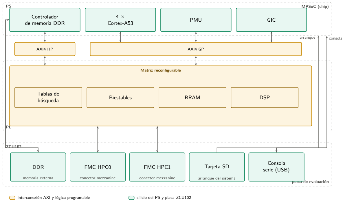
Figura 2.1: MPSoC Zynq UltraScale+ y entorno de la ZCU102.
