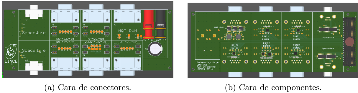
Figura 3.13: Render 3D de la revisión V2 de la placa AOCs.
