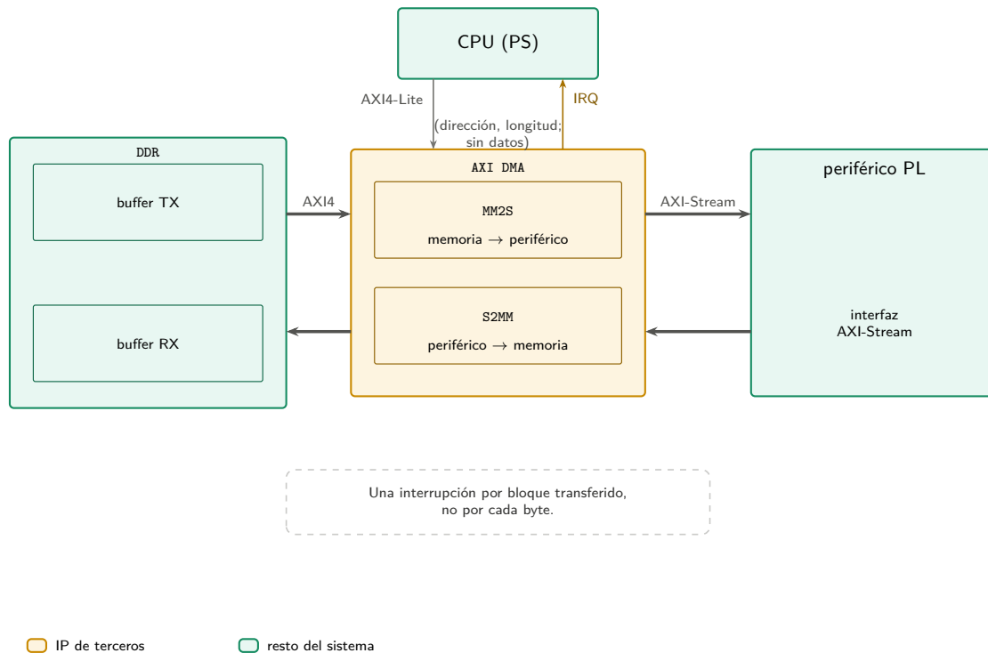
Figura 2.4: Transferencia por acceso directo a memoria.
