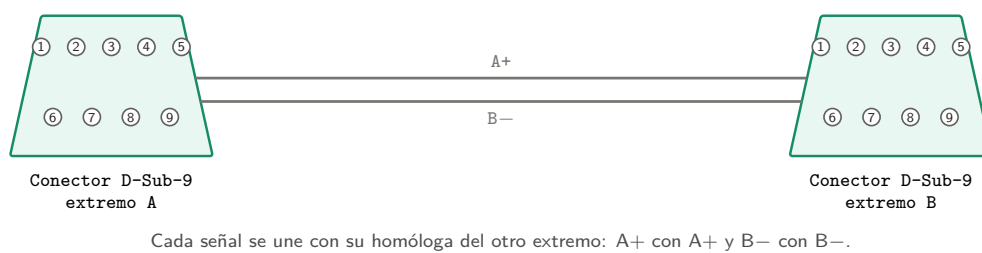
Figura 3.19: Arnés de loopback RS485 a 2 hilos entre dos conectores D-Sub-9.
