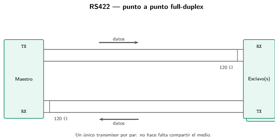
Figura 2.2: Topologías RS485 y RS422.
