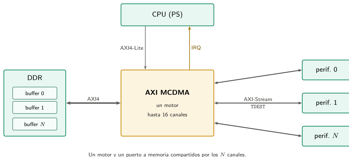
Figura 2.7: Transferencia multicanal con AXI MCDMA.
