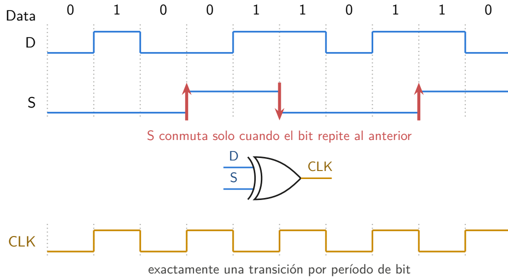
Figura 2.4: Codificación Data-Strobe y recuperación del reloj.
