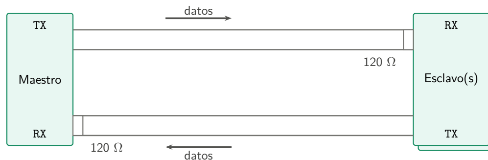
Figura 2.2: Topologías RS485 y RS422.
