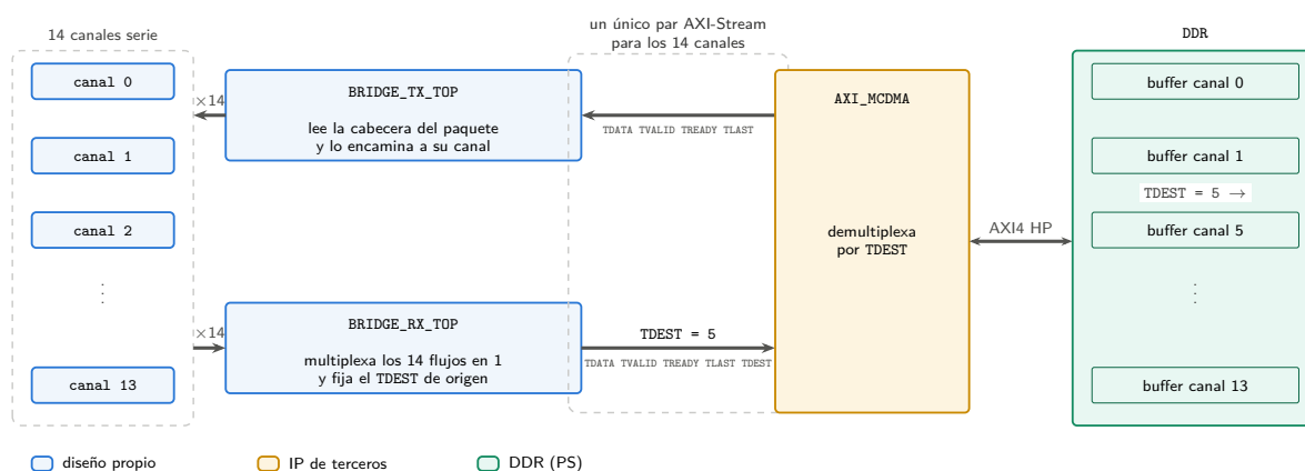
Figura 3.18: Multiplexado de los catorce canales por TDEST.
