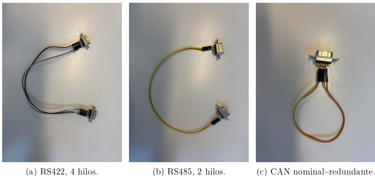
Figura 3.16: Arneses de loopback sobre conector D-Sub-9.
