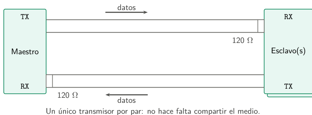
Figura 2.2: Topologías RS485 y RS422.
