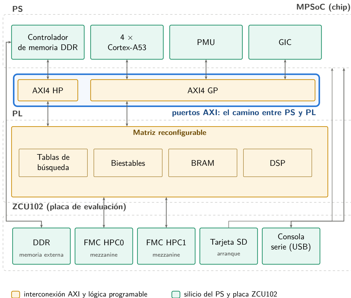
Figura 2.1: Reparto PS–PL del MPSoC y entorno de la ZCU102.
