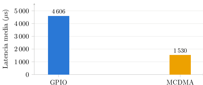
Figura 4.12: Latencia media de entrega de un frame de 11 bytes.
