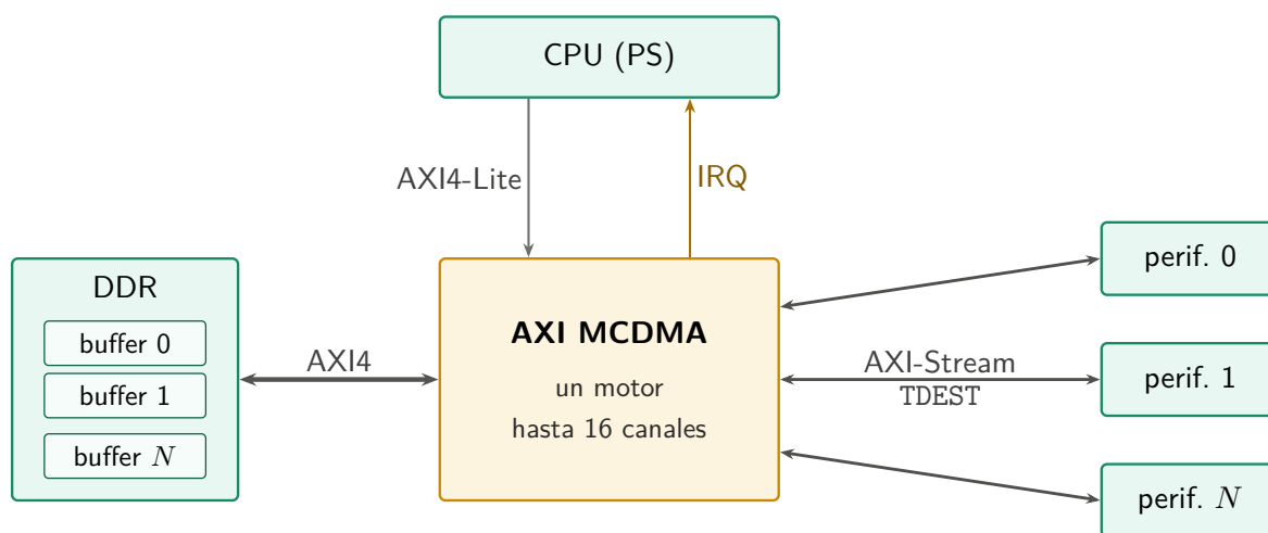
Figura 2.7: Transferencia multicanal con AXI MCDMA.
