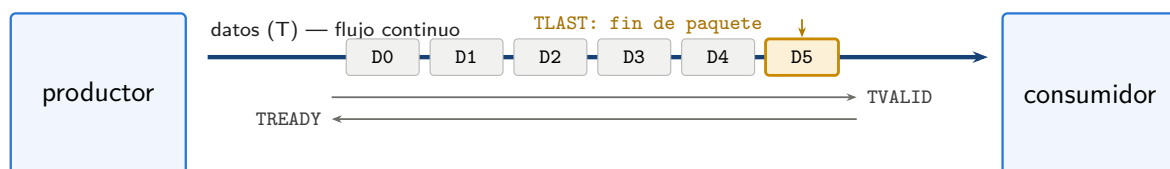
Figura 2.5: Único canal de un enlace AXI4-Stream.
