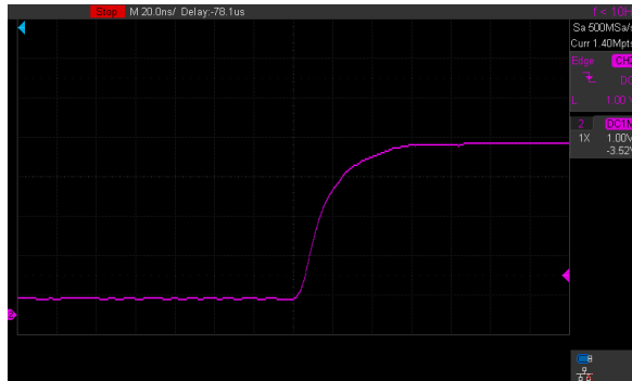
(a) Subida sin limitador (20 ns/div).
