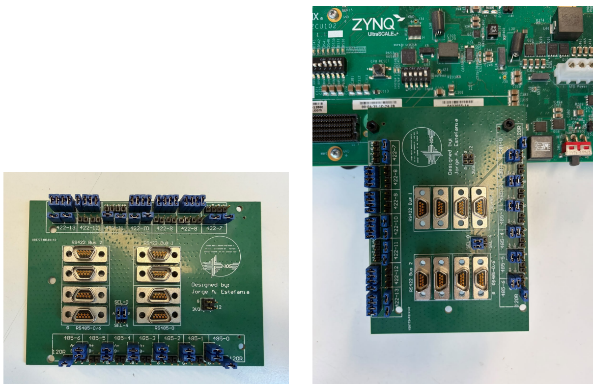
(a) Vista superior: conectores D-Sub-9 y jumpers de topología.
