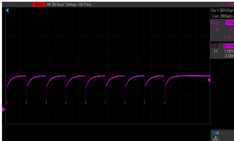
Figura 4.6: Señal diferencial CAN sin resistencias de terminación.
