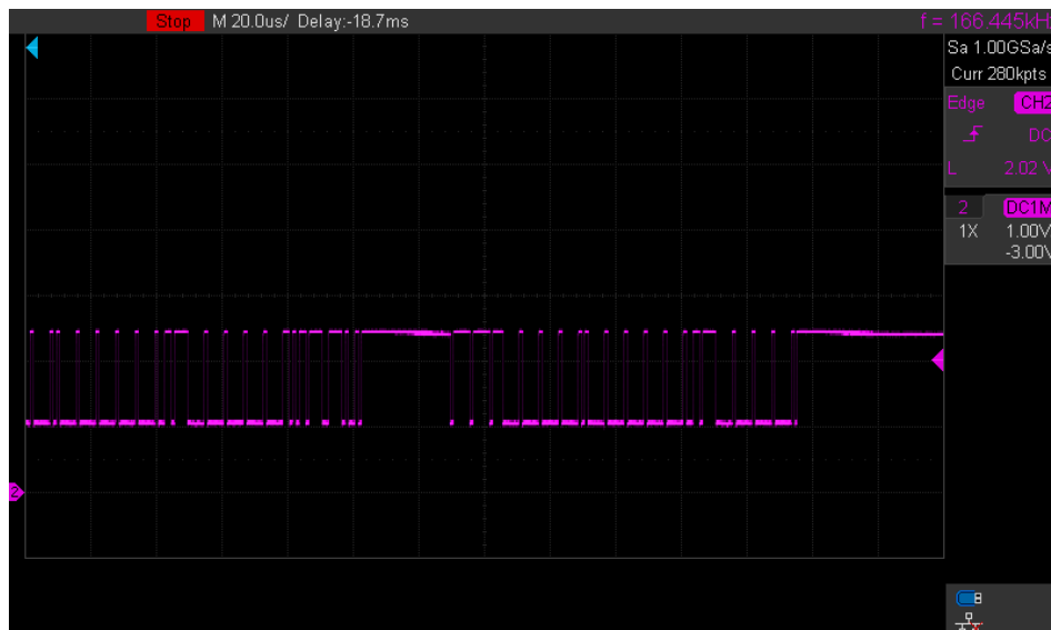
Figura 4.7: Señal diferencial CAN con resistencias de terminación ( 60\ \Omega + 60\ \Omega ).
