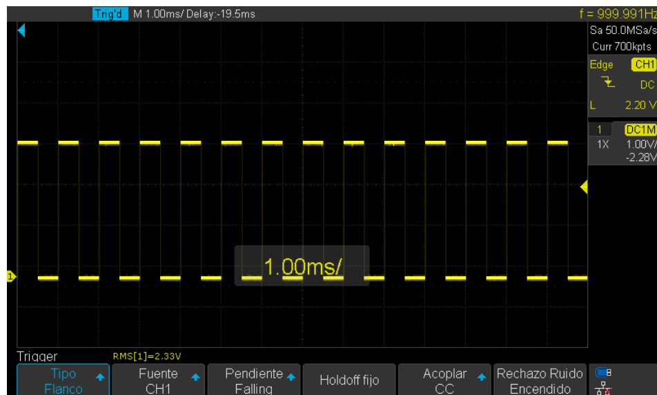
Figura 4.9: Señal PWM medida en el conector J5 de la placa CDHS: canal de 1 kHz con duty cycle del 50 %.
