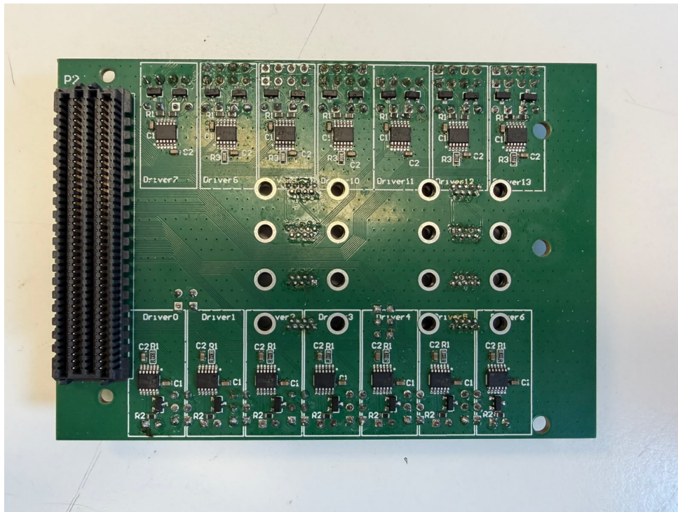
Figura 3.4: Arquitectura general de la placa de comunicación serie: los siete drivers RS422 (Driver7–Driver13, arriba), el conector FMC (P2, izquierda) y los siete drivers RS485 (Driver0–Driver6, abajo).
