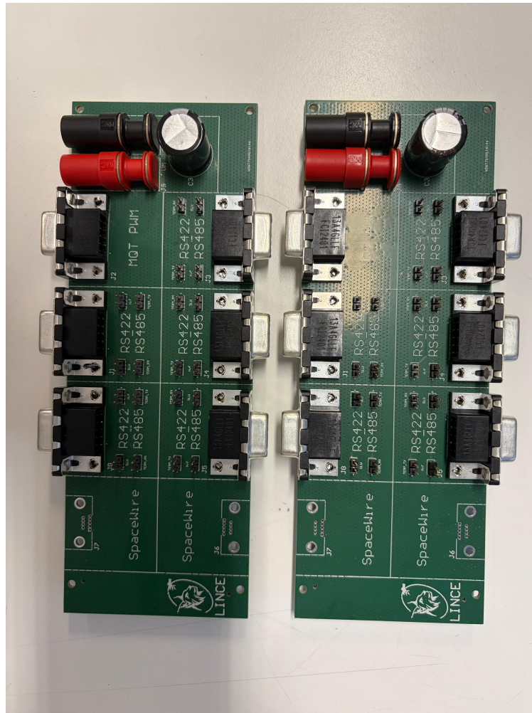
Figura 4.3: Placas AOCS con componentes montados (vista superior de las dos unidades fabricadas).
