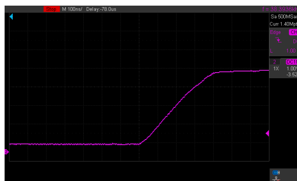
(b) Subida con limitador (100 ns/div).
