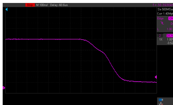
(d) Bajada con limitador (100 ns/div).
