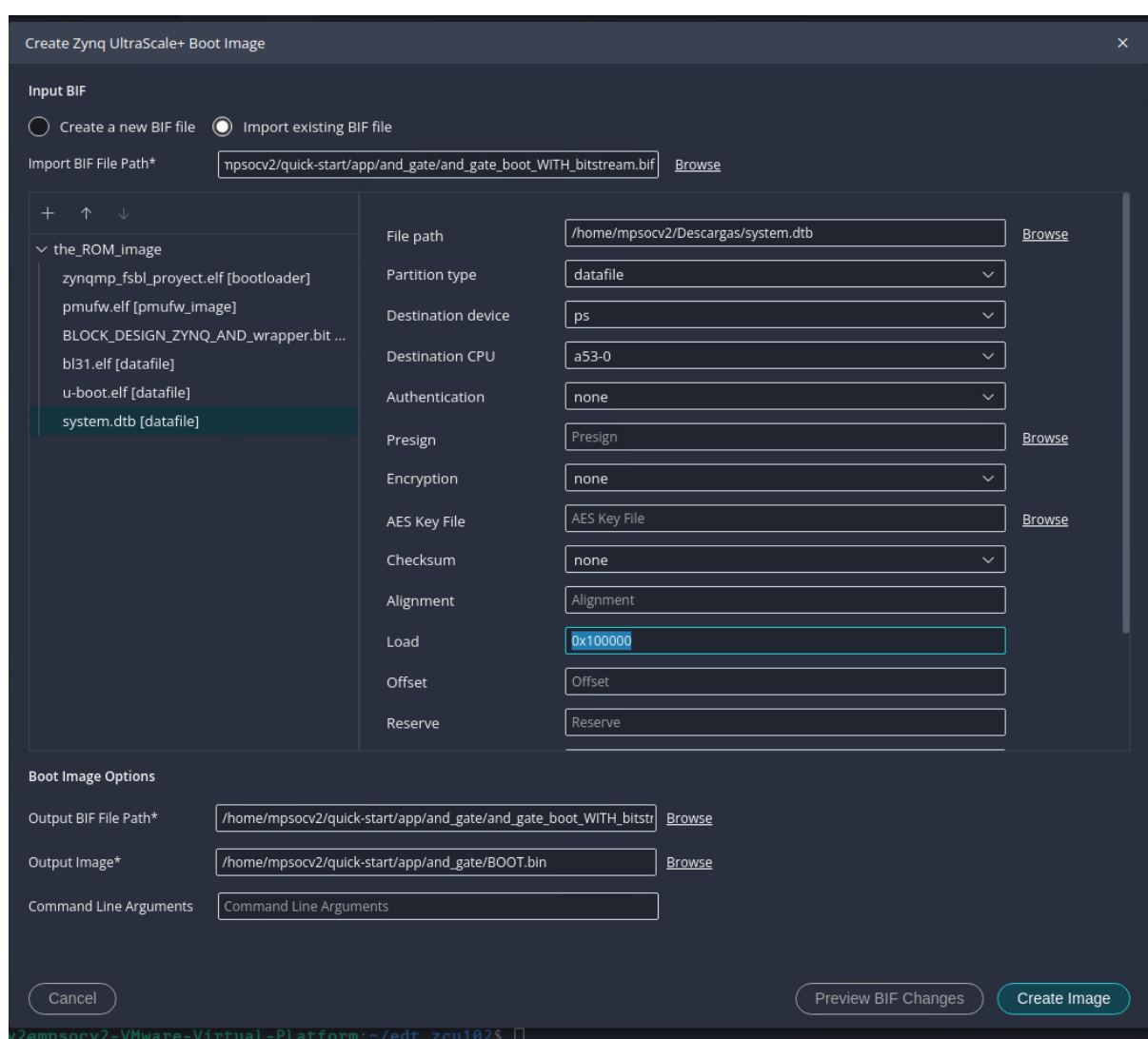
Figura 3.2: Generador de imágenes de arranque de Vitis.
