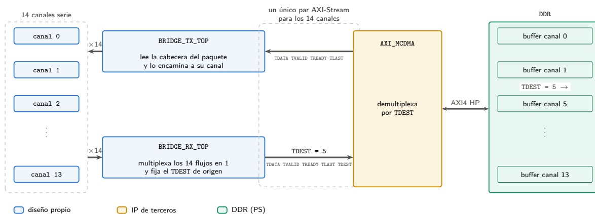
Figura 3.20: Multiplexado de los catorce canales por TDEST .
