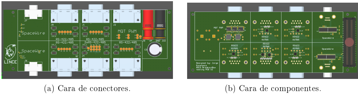
Figura 3.11: Render 3D de la revisión V2 de la placa AOCs.
