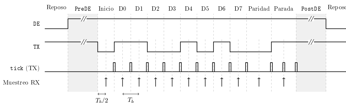
Figura 3.3: Cronograma de una trama completa en configuración 8E1, LSB first .
