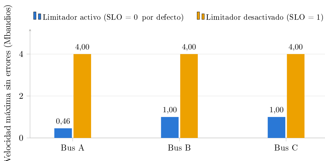
Figura 4.9: Velocidad máxima sin errores en cada bus según el valor del bit SLO.
