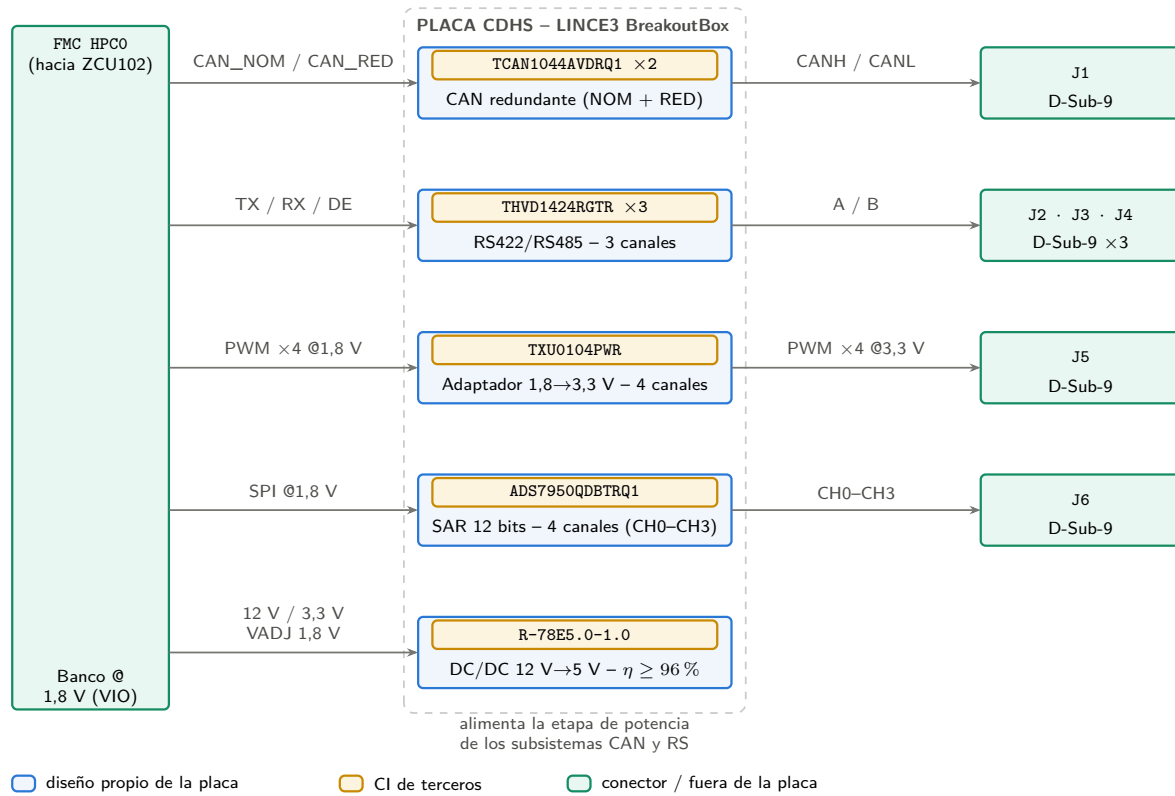
Figura 3.8: Diagrama de bloques de la placa CDHS.
