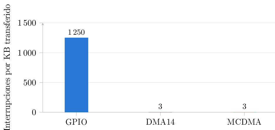
Figura 4.12: Interrupciones por kilobyte transferido, por variante.
