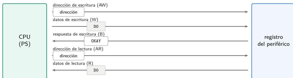
Figura 2.3: Canales de una transacción AXI4-Lite.
