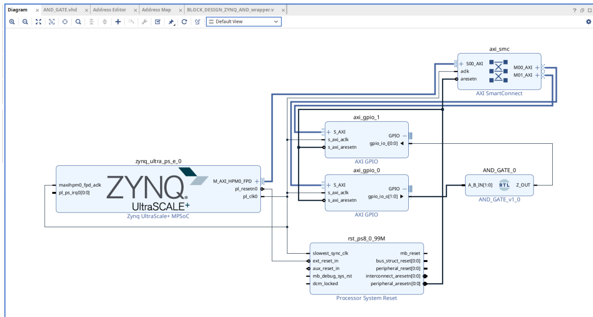
Figura 3.1: Block Design del ejemplo de la puerta AND.
