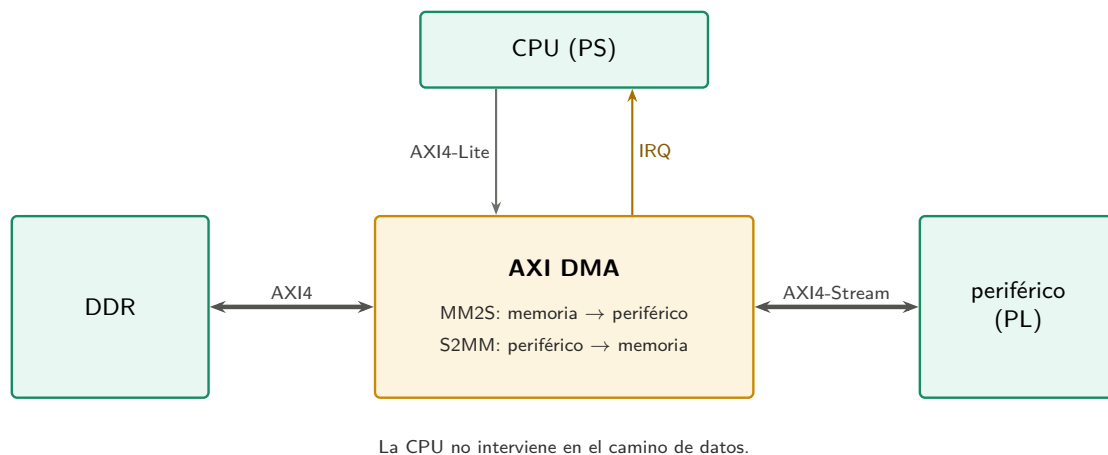
Figura 2.6: Transferencia por acceso directo a memoria.
