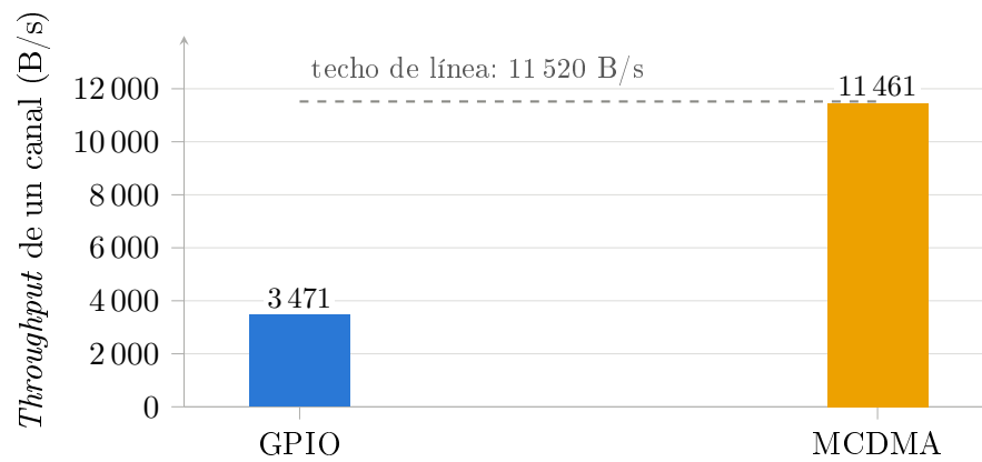
Figura 4.14: Throughput de un canal frente al techo físico de la línea.
