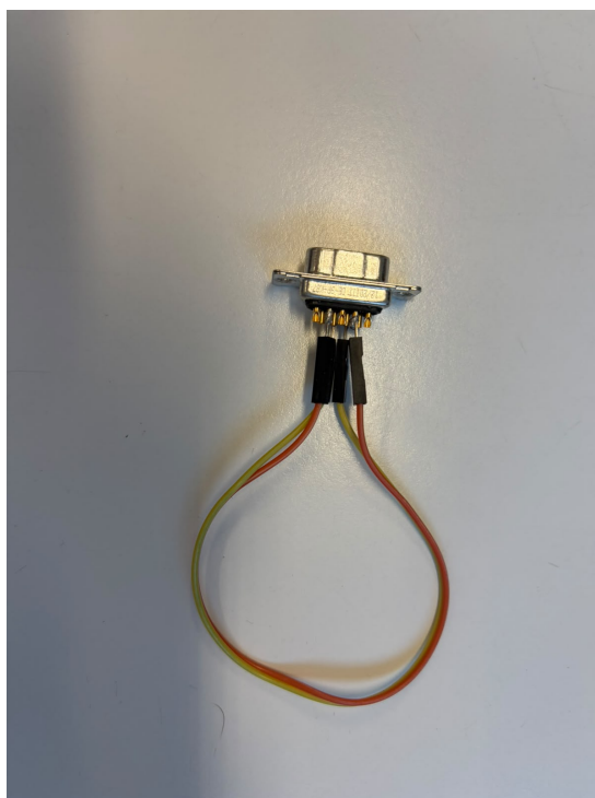
Figura 3.20: Arnés de interconexión CAN nominal–redundante.
