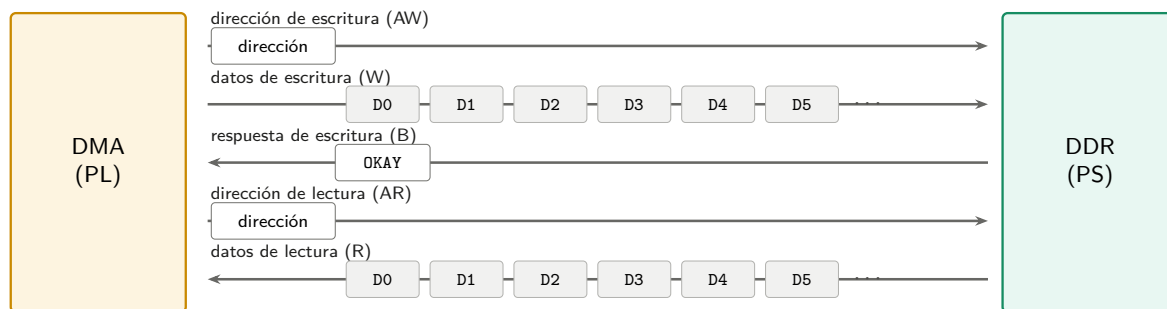
Figura 2.4: Canales de una transacción AXI4 full.
