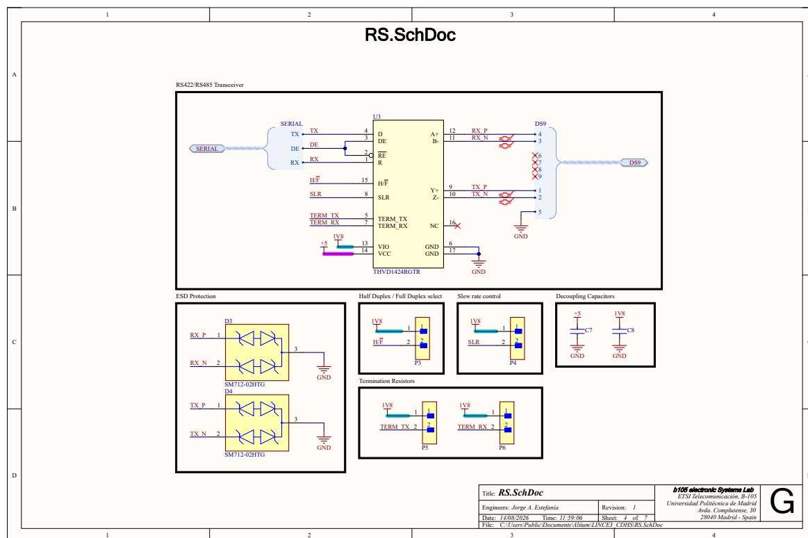
Figura 3.11: Canal RS de la placa CDHS con el THVD1424RGTR.
