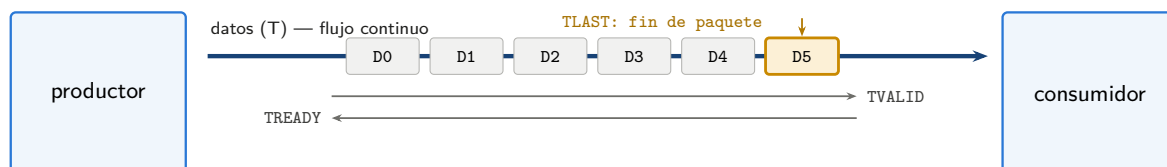
Figura 2.5: Único canal de un enlace AXI4-Stream.
