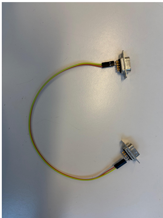
Figura 3.19: Arnés de loopback RS485 a 2 hilos entre dos conectores D-Sub-9.
