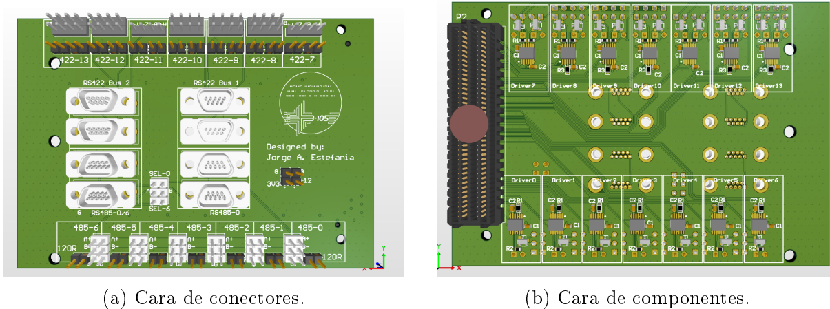
Figura 3.7: Render 3D de la placa de comunicación serie.
