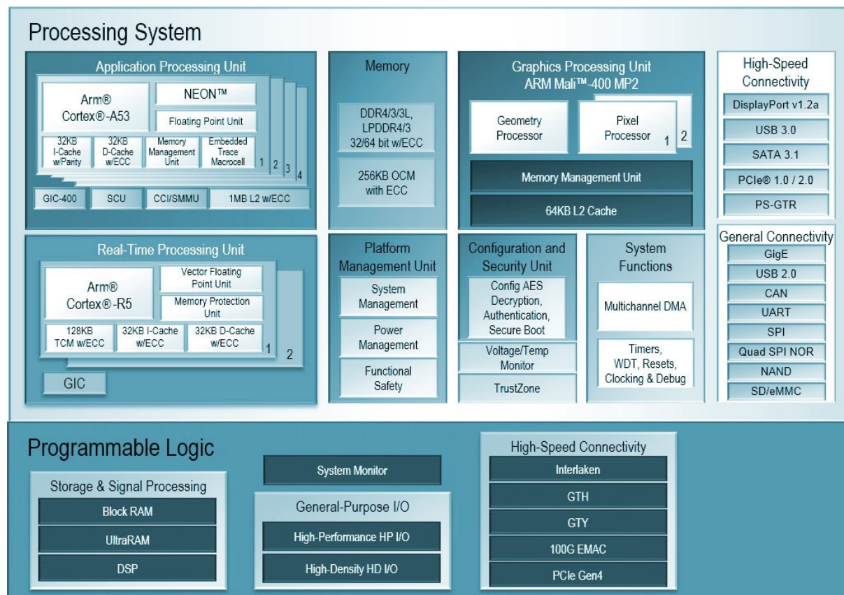
Figura 2.1: Arquitectura del MPSoC Zynq UltraScale+ (fuente: AMD).
