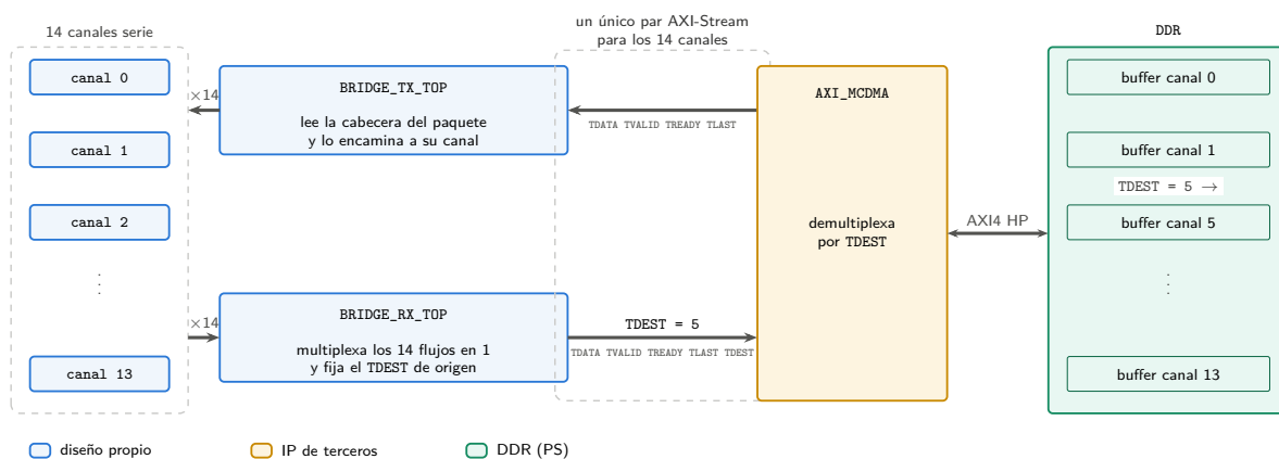
Figura 3.22: Multiplexado de los catorce canales por TDEST .
