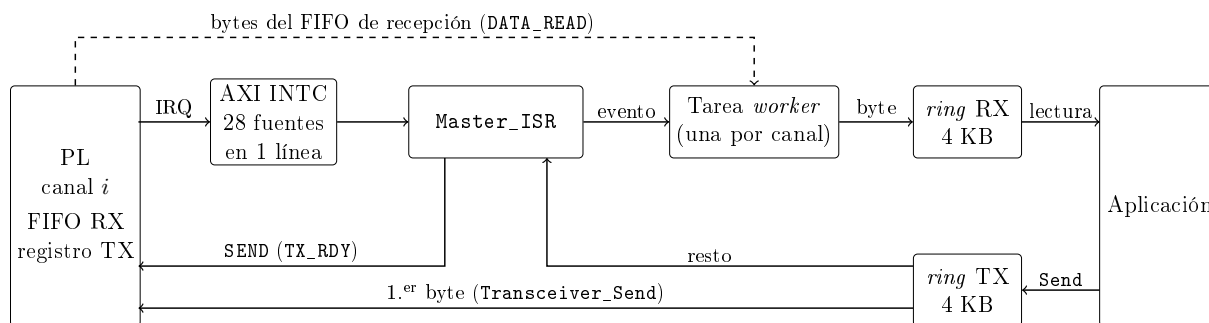
Figura 3.5: Camino de un byte entre la lógica programable y la aplicación.
