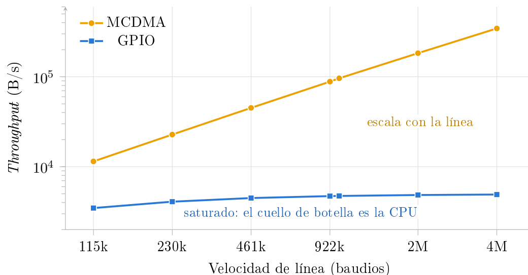
Figura 4.15: Throughput frente a la velocidad de línea, en escala logarítmica.
