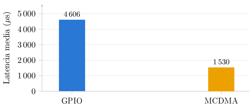
Figura 4.13: Latencia media de entrega de un frame de 11 bytes.
