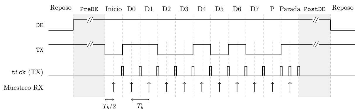
Figura 3.4: Cronograma de una trama completa, con la configuración 8 bits de datos, paridad par, un bit de parada y orden LSB first (dato 0x53). El transmisor consume un tick por frontera de bit y pasa al doble de frecuencia en el campo de parada, donde cuenta semiperiodos. El receptor, tras alinear su fase medio bit después del flanco de inicio, muestrea en el centro de cada bit; el primer muestreo, en el centro del bit de inicio, es el que descarta los falsos inicios de trama. Las zonas sombreadas PreDE y PostDE no están a escala: duran 100 \mu s frente a los 8,7 \mu s del tiempo de bit a 115 200 baudios.
