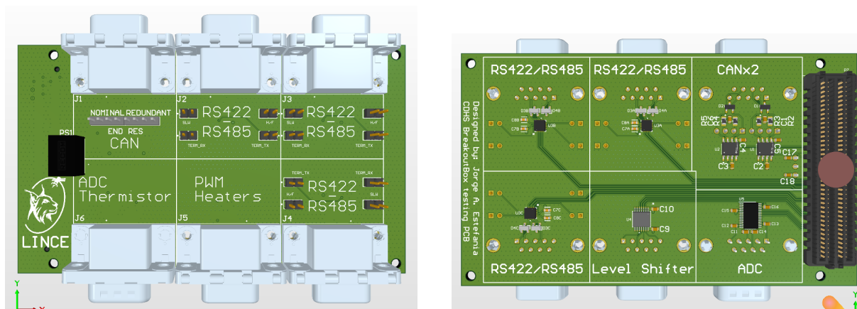
(a) Cara de conectores: los seis D-Sub-9 (J1–J6), los jumpers de terminación del CAN y los de configuración H/F, SLR y terminación de los tres canales RS, con el módulo DC/DC PS1 en el borde izquierdo.
