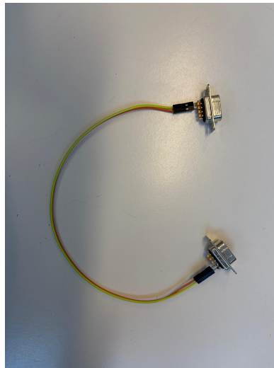
(b) RS485, 2 hilos.
