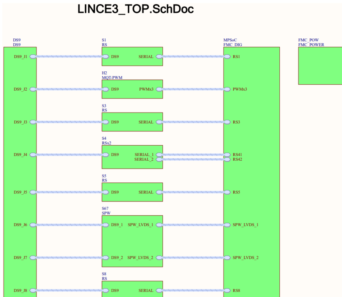
Figura 4.7: Hoja de nivel superior del esquema de la placa AOCs.
