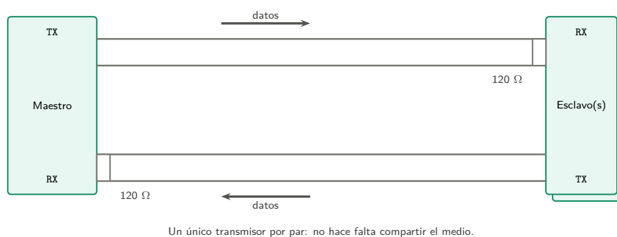
Figura 2.2: Topologías RS485 y RS422.
