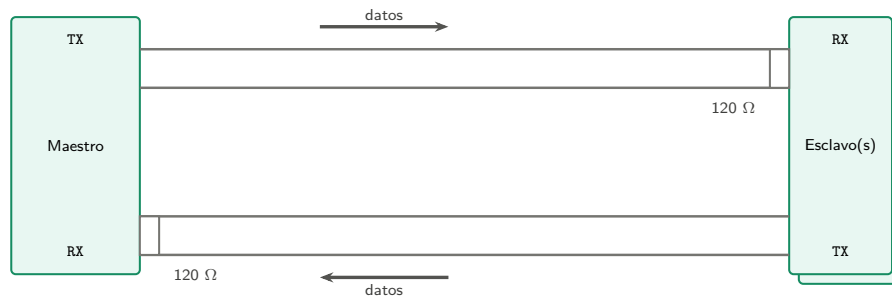
Figura 2.2: Topologías RS485 y RS422.
