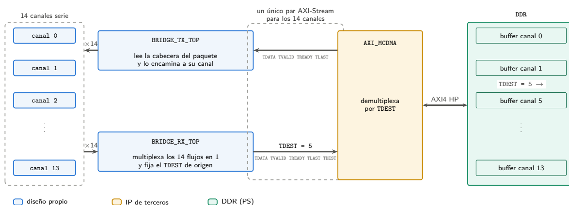
Figura 3.5: Multiplexado de los catorce canales por TDEST.
