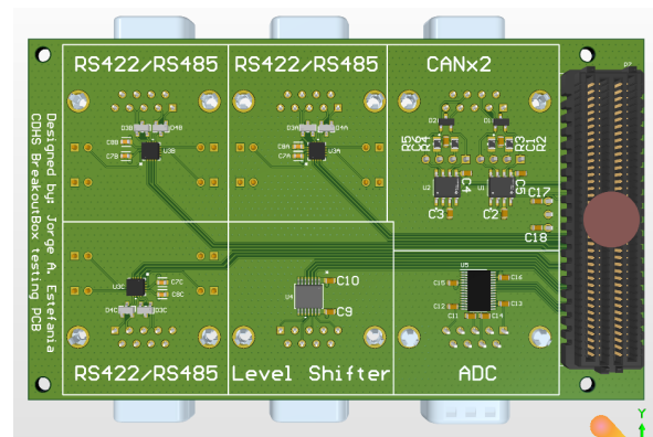
(b) Cara de componentes.
