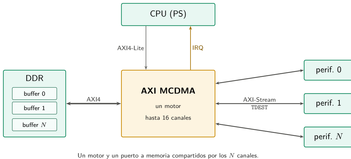
Figura 2.8: Transferencia multicanal con AXI MCDMA.
