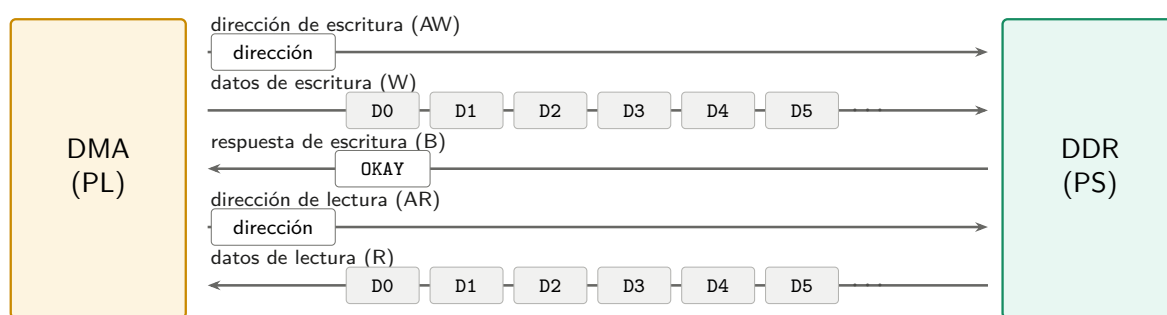
Figura 2.5: Canales de una transacción AXI4 full.
