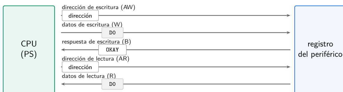
Figura 2.4: Canales de una transacción AXI4-Lite.
