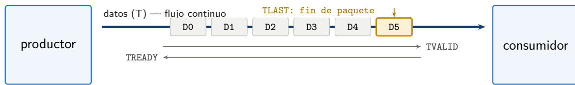
Figura 2.6: Único canal de un enlace AXI4-Stream.
