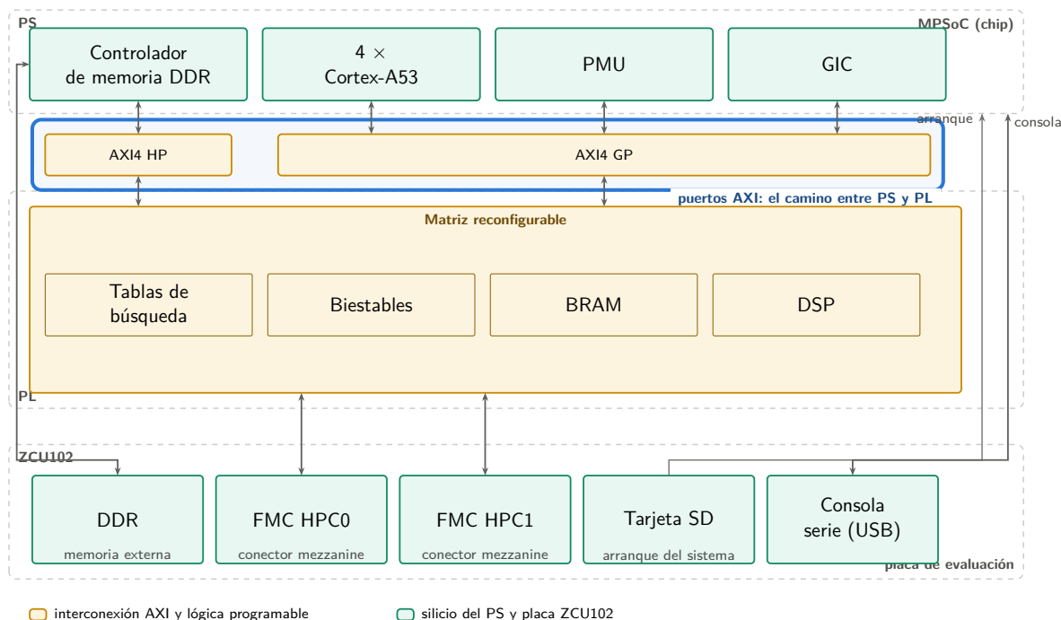
Figura 2.1: Reparto PS-PL del MPSoC y entorno de la ZCU102.
