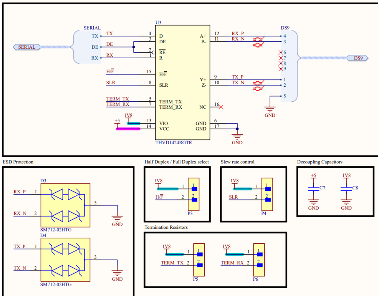
Figura 3.9: Canal RS de la placa CDHS con el THVD1424RGTR.
