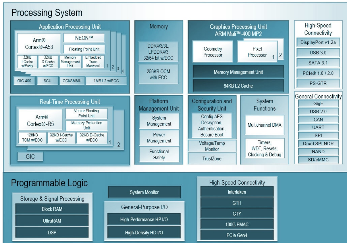
Figura 2.2: Arquitectura del MPSoC Zynq UltraScale+ (fuente: AMD).
