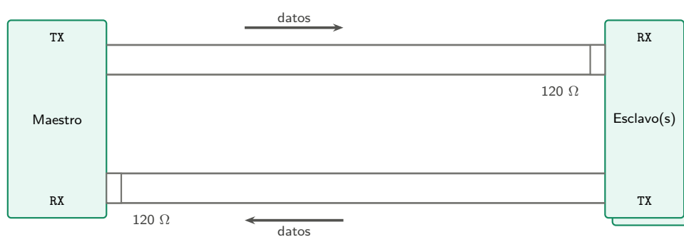
Figura 2.3: Topologías RS485 y RS422.
