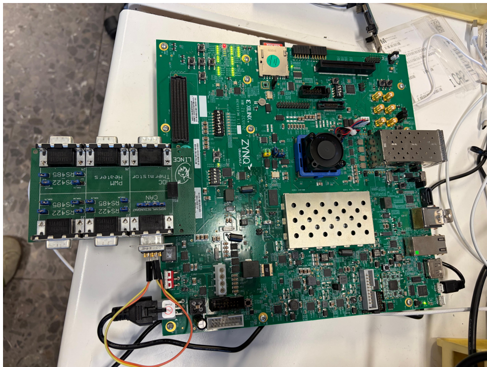
Figura 4.1: Sistema completo montado: ZCU102 con la placa CDHS conectada al FMC.
