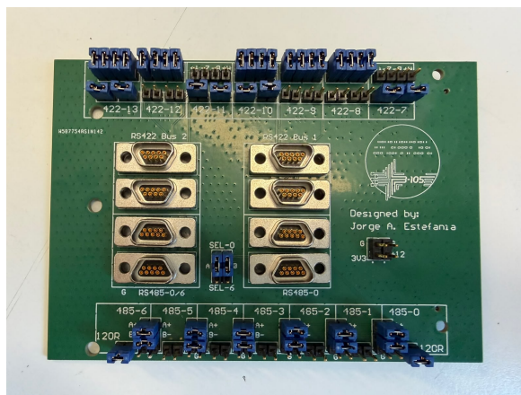
(a) Vista superior: conectores D-Sub-9 y jum- pers de topología.
