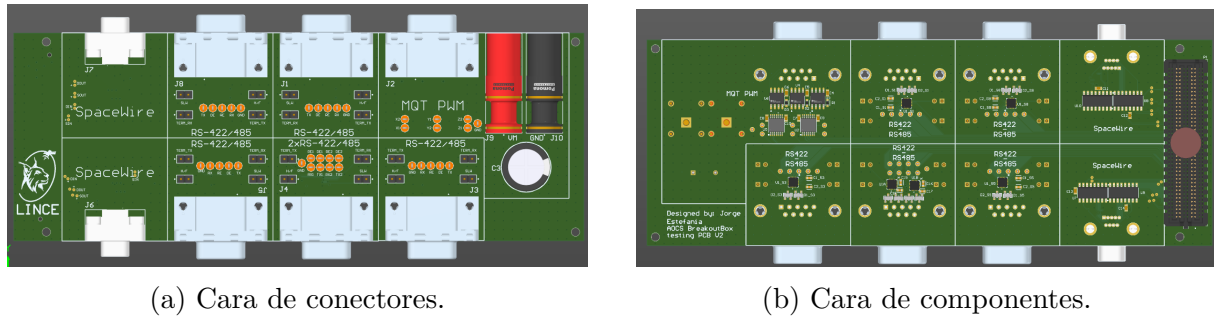
Figura 4.8: Render 3D de la revisión V2 de la placa AOCs.
