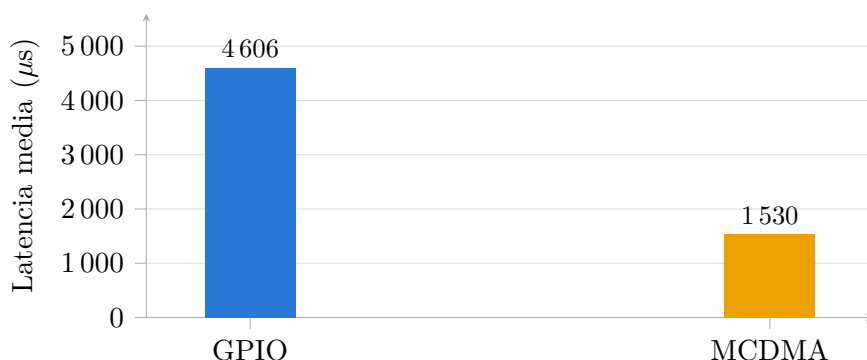
Figura 5.12: Latencia media de entrega de un frame de 11 bytes.
