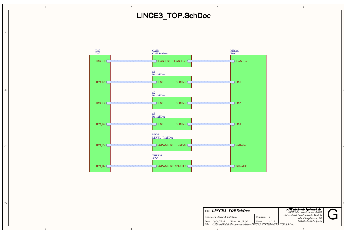
Figura 3.6: Hoja de nivel superior del esquemático de la placa CDHS.
