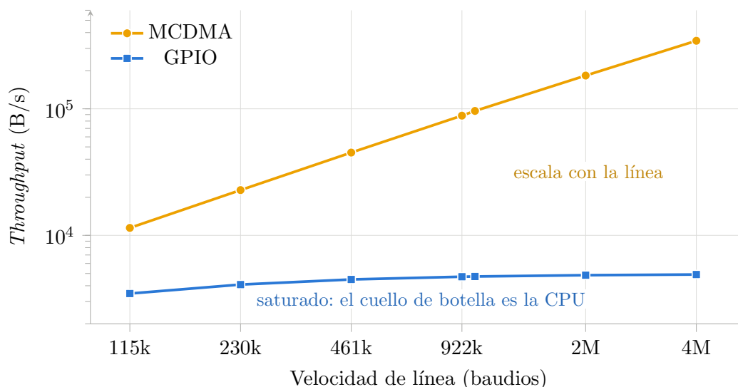
Figura 4.12: Throughput frente a la velocidad de línea, en escala logarítmica.
