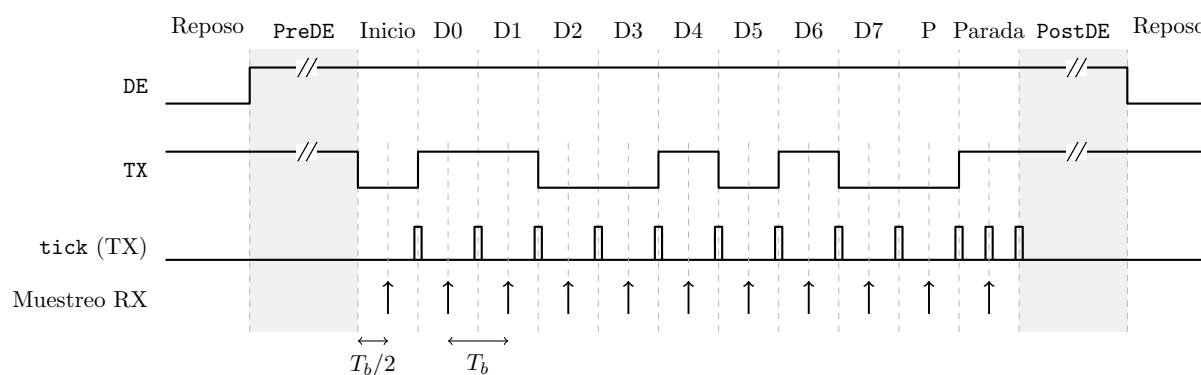
Figura 3.3: Cronograma de una trama completa en configuración 8E1, LSB first .
