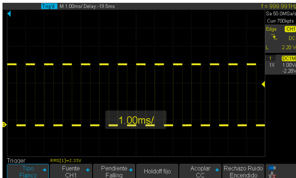
Figura 4.5: Señal PWM en el conector J5 de la placa CDHS (1 kHz, 50 %).
