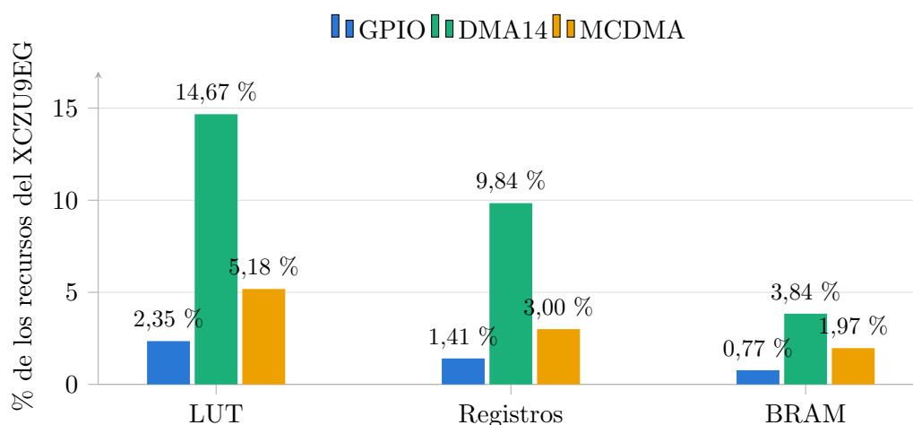
Figura 4.8: Ocupación de la FPGA por variante.
