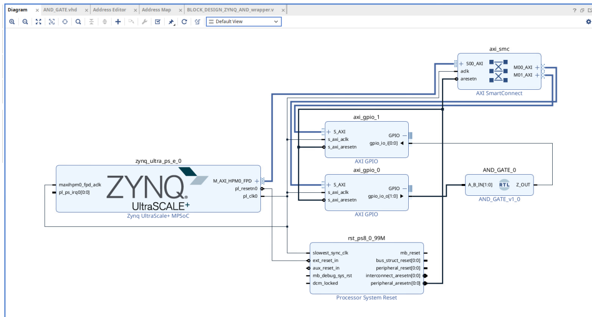
Figura 3.1: Block Design del ejemplo de la puerta AND.
