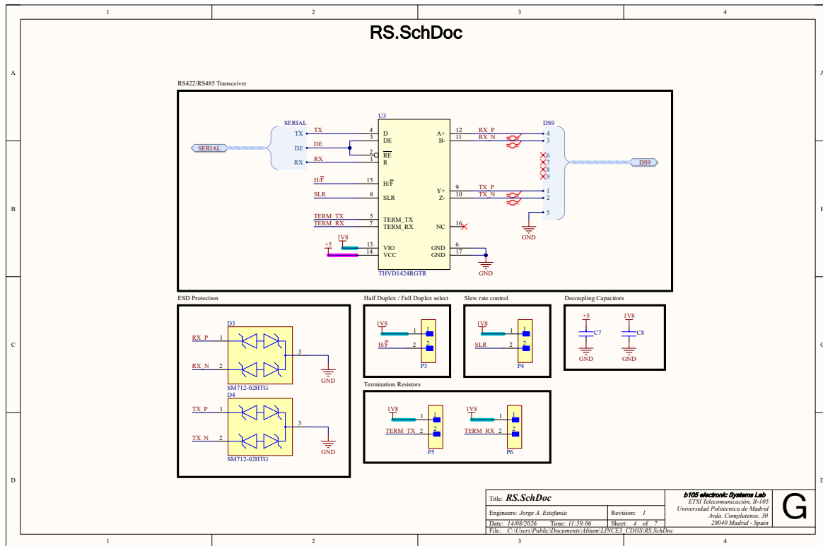
Figura 3.9: Canal RS de la placa CDHS con el THVD1424RGTR.
