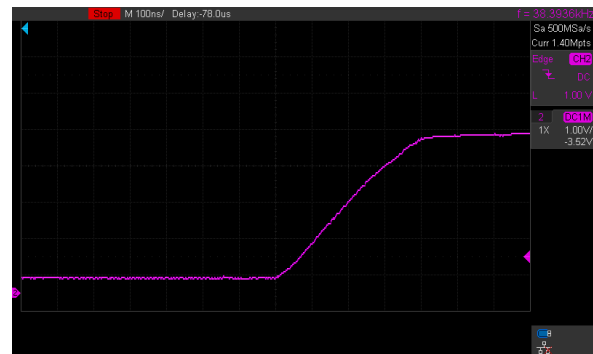
(b) Subida con limitador (100 ns/div).
