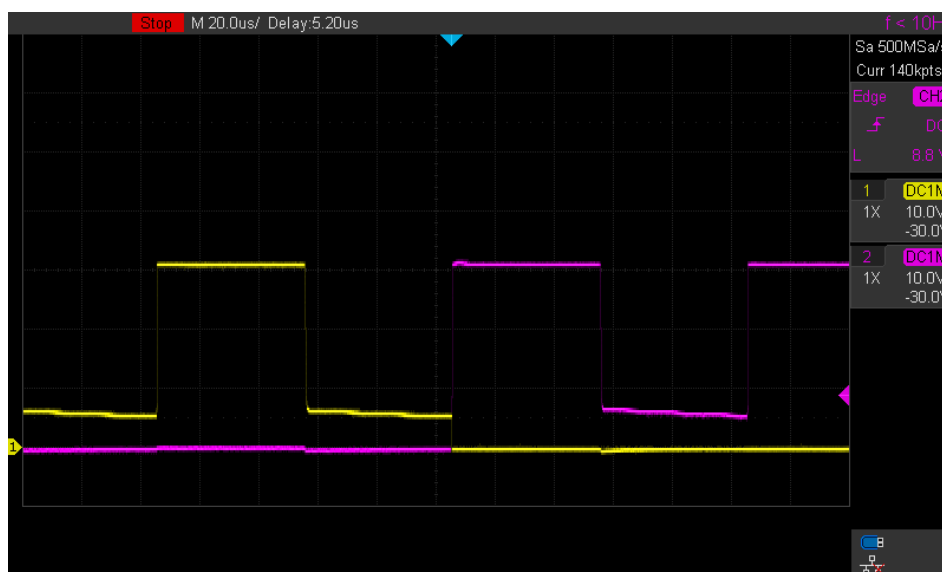
Figura 4.7: Señales PWM de control de motor en la placa AOCS.
