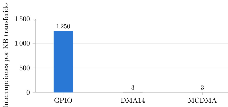
Figura 4.9: Interrupciones por kilobyte transferido, por variante.
