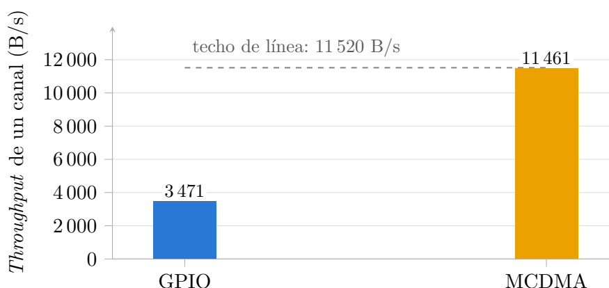
Figura 4.11: Throughput de un canal frente al techo físico de la línea.
