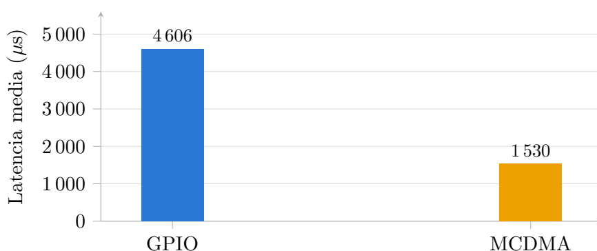
Figura 4.10: Latencia media de entrega de un frame de 11 bytes.
