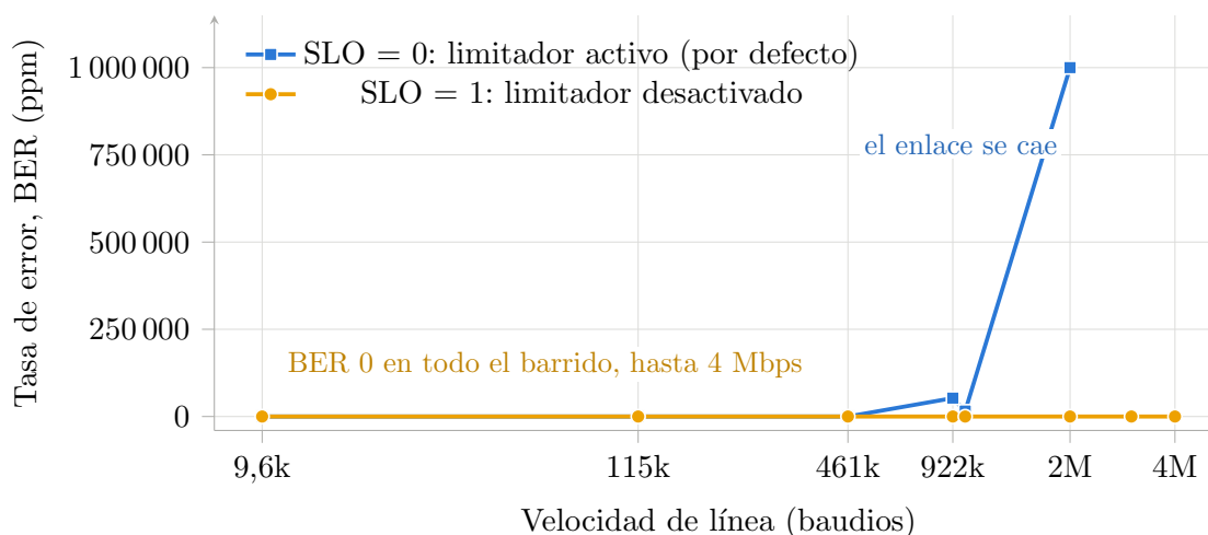
Figura 4.15: Tasa de error del bus multipunto frente a la velocidad, con y sin limitador de slew .
