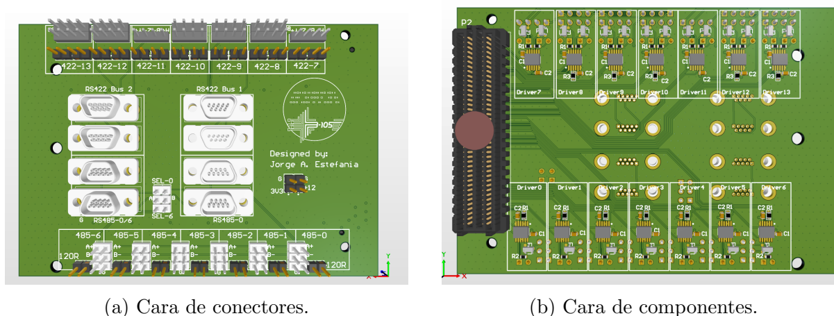
Figura 3.7: Render 3D de la placa de comunicación serie.
