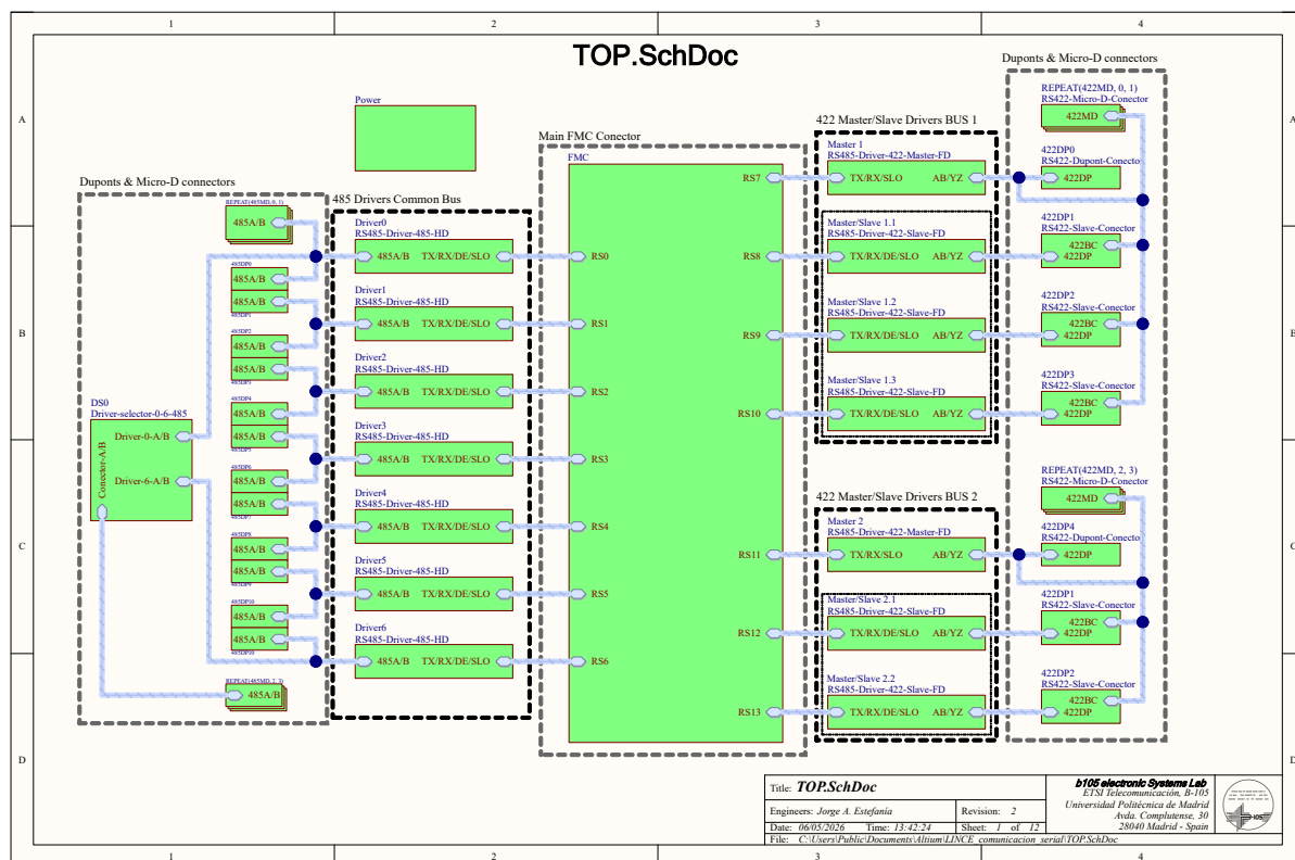
Figura 3.6: Hoja de nivel superior del esquemático de la placa de comunicación serie.
