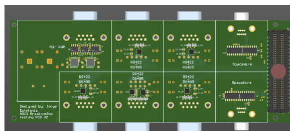
(b) Cara de componentes: los transeptores THVD1424RGTR de los canales RS, los repetidores LVDS de SpaceWire, la etapa de motores y el conector FMC (P1).
