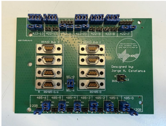
(a) Vista superior de la placa.
