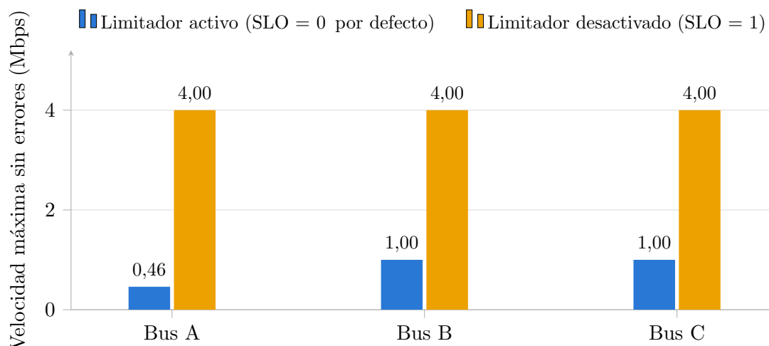
Figura 4.9: Velocidad máxima sin errores en cada bus según el valor del bit SLO.
