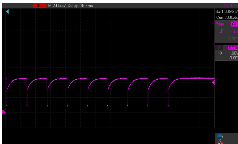
Figura 4.3: Señal diferencial CAN sin resistencias de terminación.
