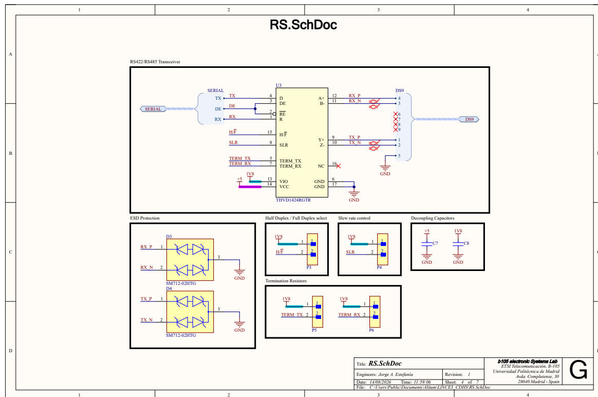
Figura 3.10: Canal RS de la placa CDHS con el THVD1424RGTR.
