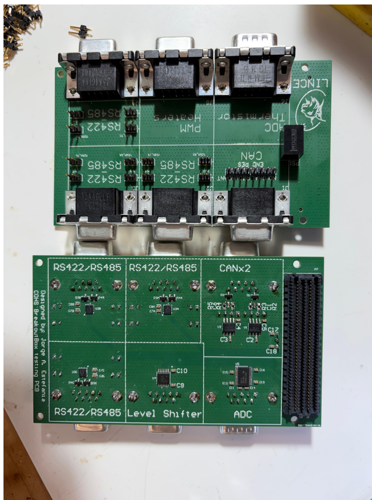
Figura 3.14: Placa CDHS tras el proceso de soldadura.
