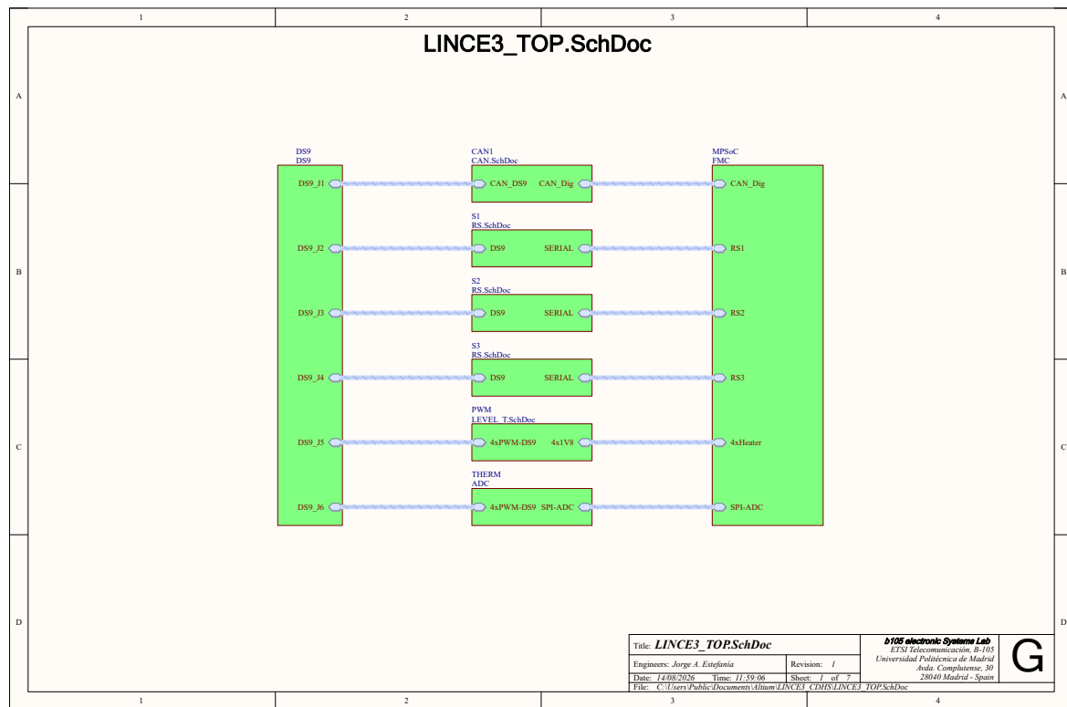
Figura 3.7: Hoja de nivel superior del esquemático de la placa CDHS.
