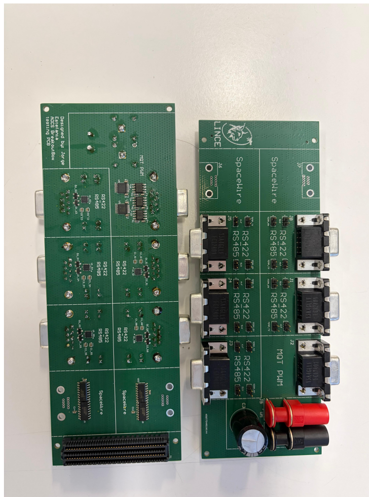
Figura 3.15: Placa AOCS tras el proceso de soldadura.
