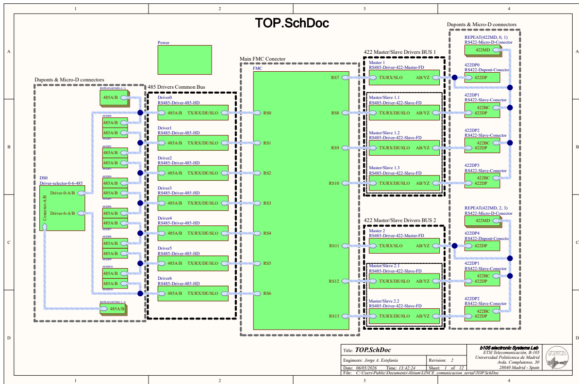
Figura 3.5: Hoja de nivel superior del esquemático de la placa de comunicación serie.
