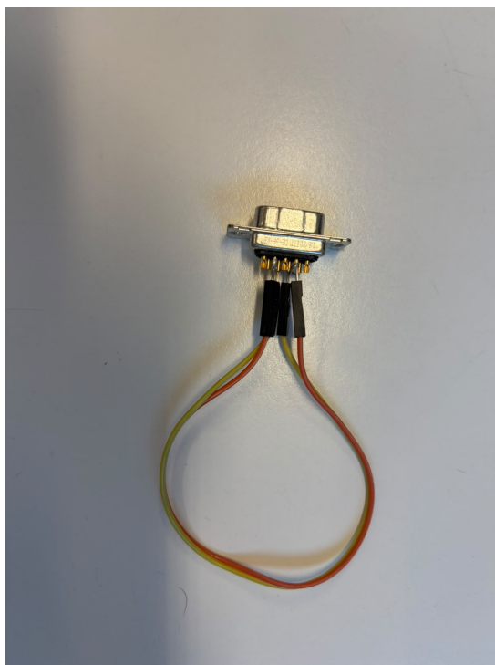
Figura 3.19: Arnés de interconexión CAN nominal–redundante.
