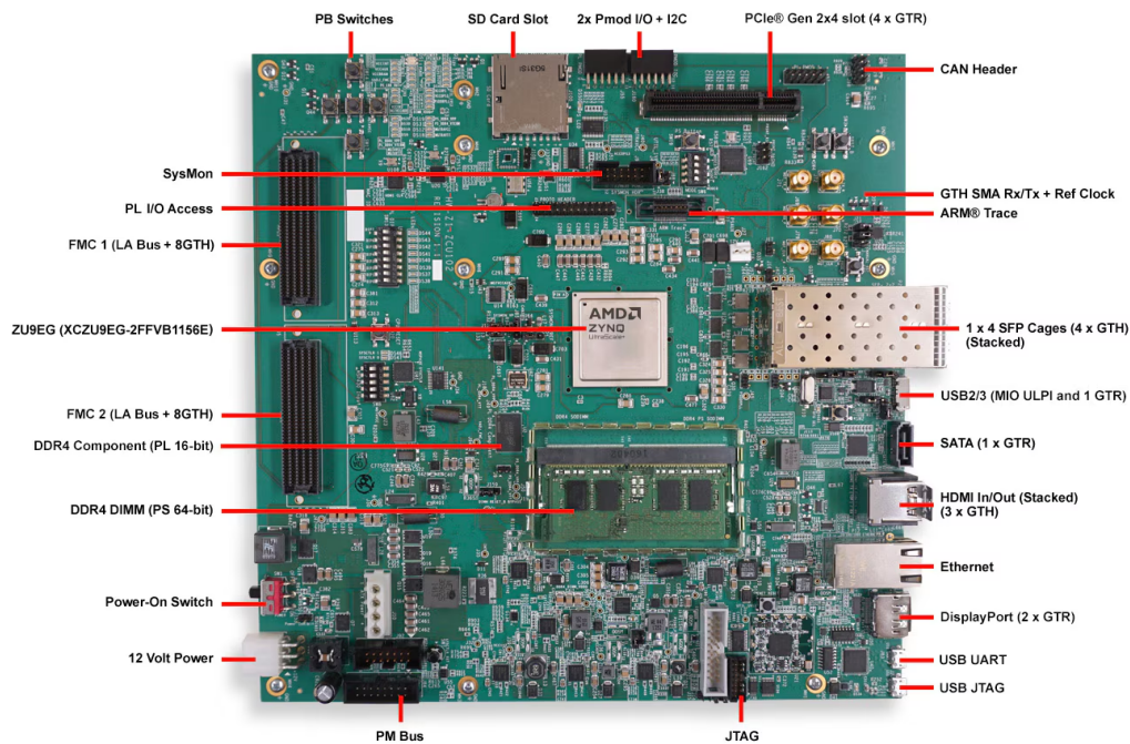
Figura 2.1: Tarjeta de evaluación ZCU102 [6].
