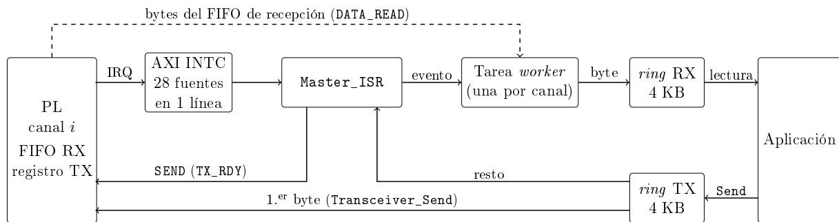
Figura 3.3: Camino de un byte entre la lógica programable y la aplicación.
