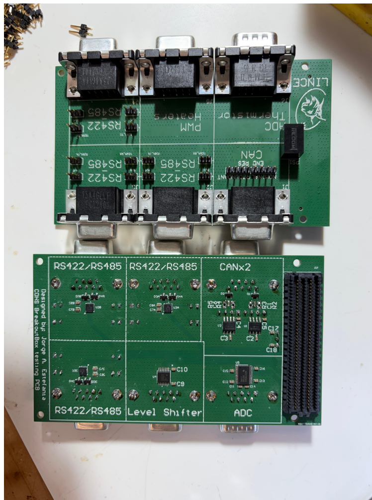
Figura 3.13: Placa CDHS tras el proceso de soldadura, con las dos caras a la vista: arriba la cara de conectores D-Sub-9 y jumbers de configuración, y abajo la cara de componentes con los transceptores, el adaptador de nivel, el ADC y el conector FMC.
