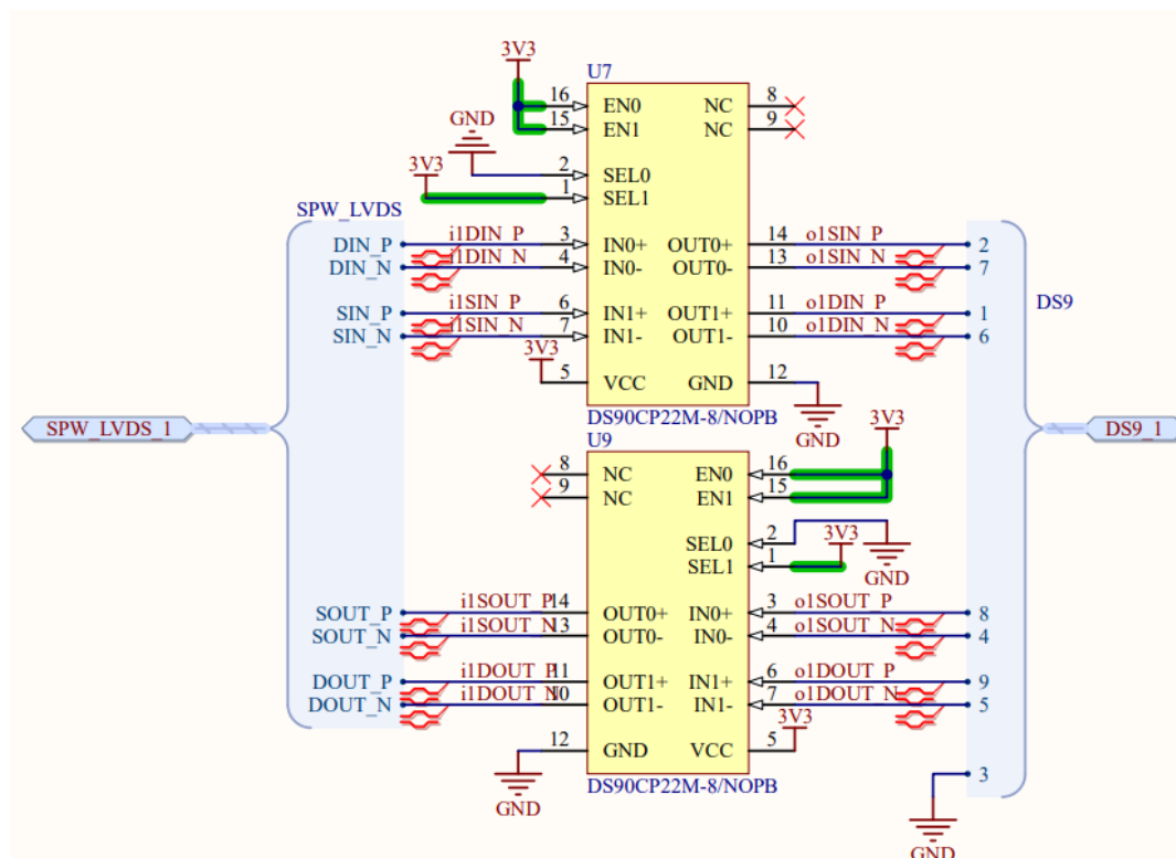
Figura 4.9: Subsistema SpaceWire de la placa AOCS.
