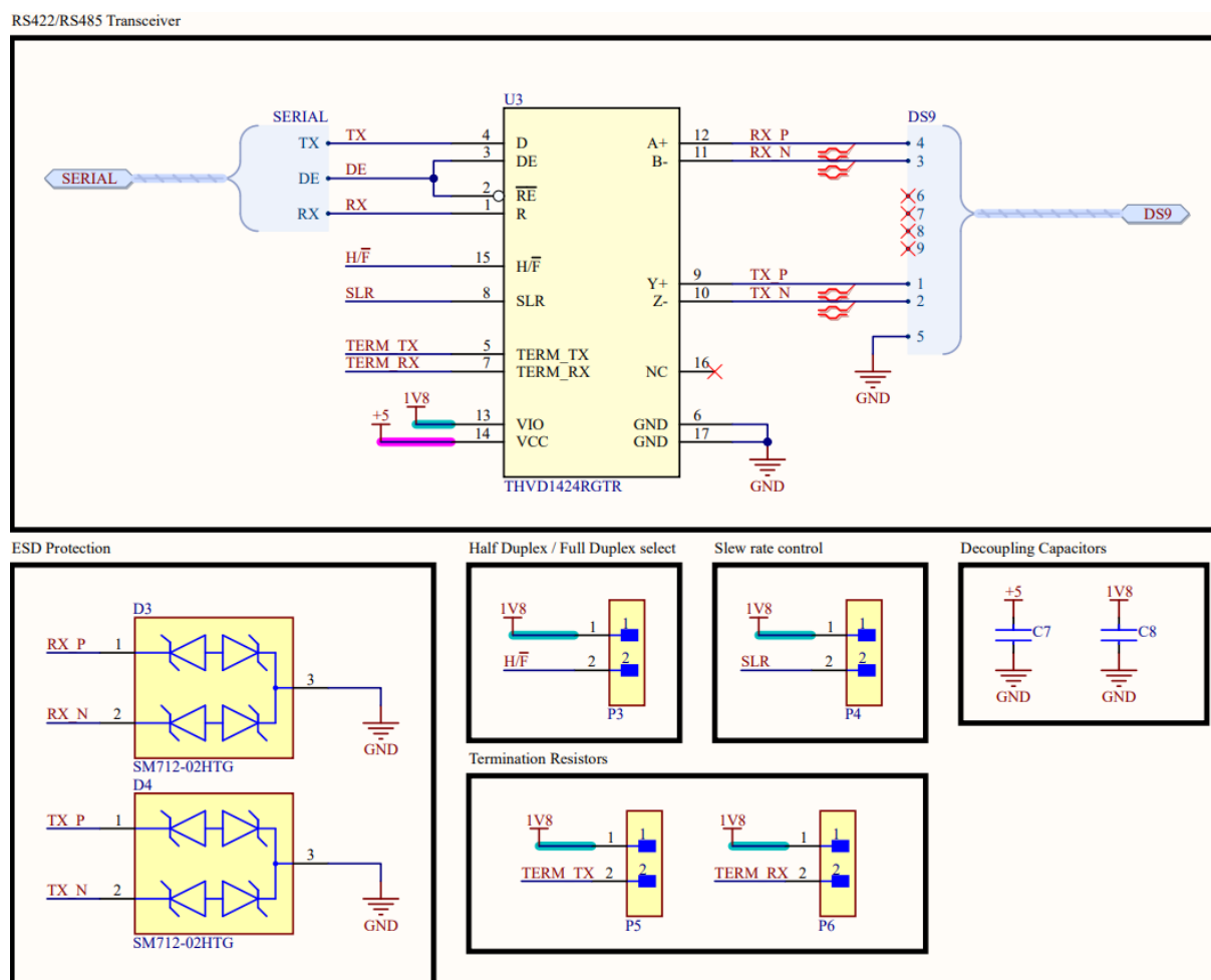
Figura 4.6: Canal RS de la placa CDHS con el THVD1424RGTR.
