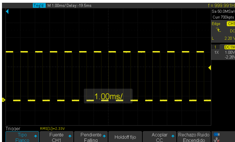
Figura 5.4: Señal PWM en el conector J5 de la placa CDHS (1 kHz, 50 %).
