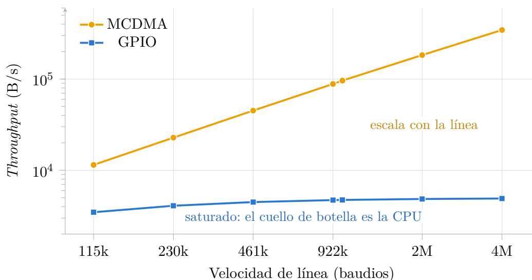
Figura 5.14: Throughput frente a la velocidad de línea, en escala logarítmica.
