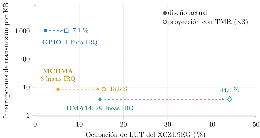
Figura 5.16: Compromiso entre ocupación y coste en interrupciones.
