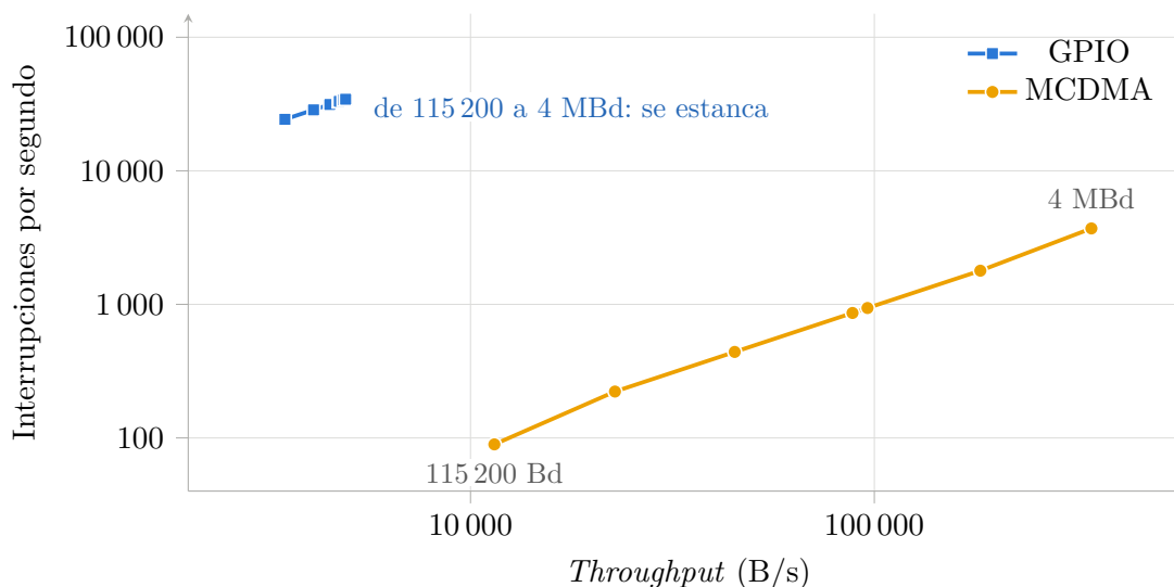
Figura 5.15: Interrupciones por segundo frente a throughput en el barrido de velocidad.
