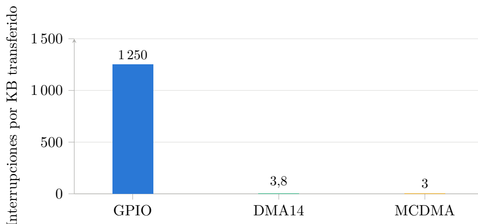
Figura 5.11: Interrupciones por kilobyte transferido, por variante.
