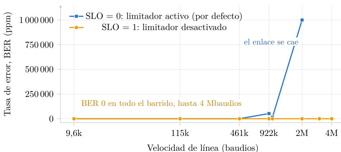
Figura 5.9: Tasa de error del bus multipunto frente a la velocidad, con y sin limitador de slew .
