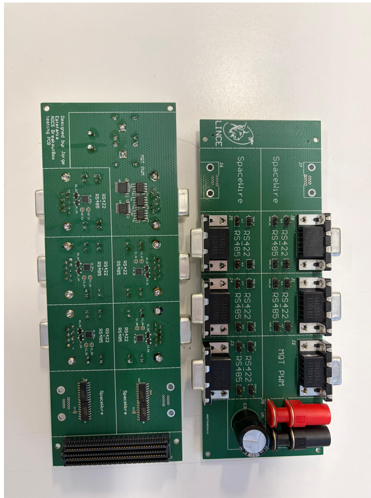
Figura 4.11: Placa AOCS tras el proceso de soldadura.
