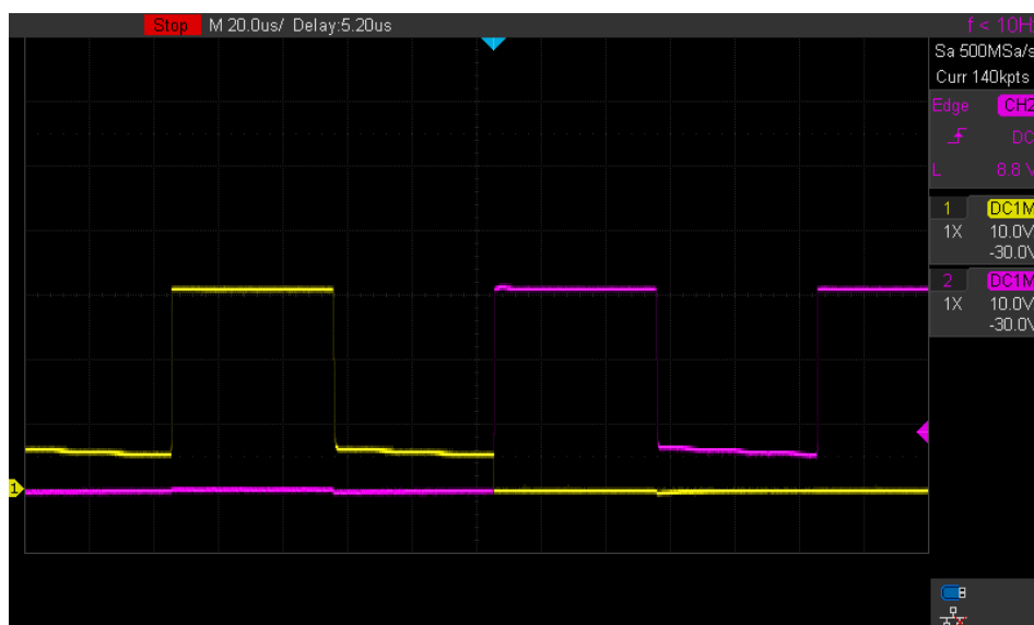
Figura 5.6: Señales PWM de control de motor en la placa AOCS.
