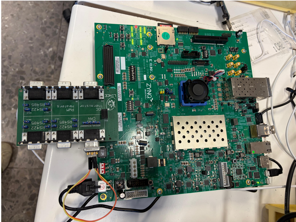
Figura 5.1: Sistema completo montado: ZCU102 con la placa CDHS.
