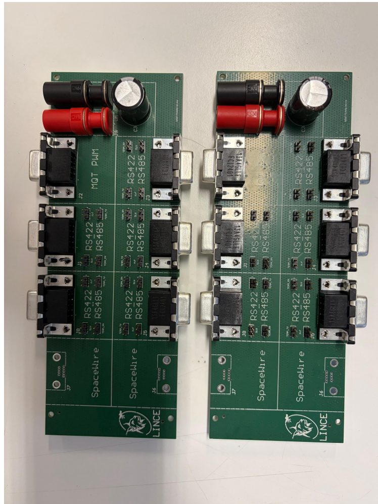
Figura 5.5: Placas AOCS con componentes montados.
