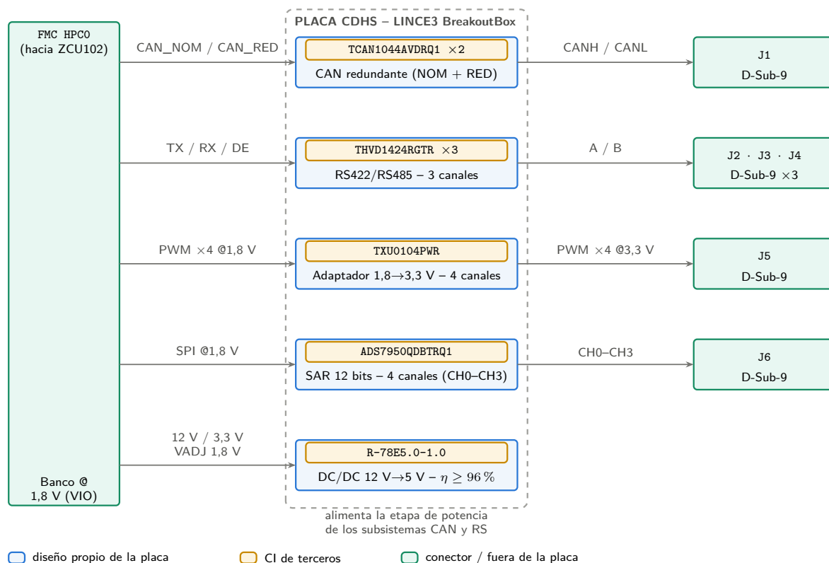
Figura 4.3: Diagrama de bloques de la placa CDHS.
