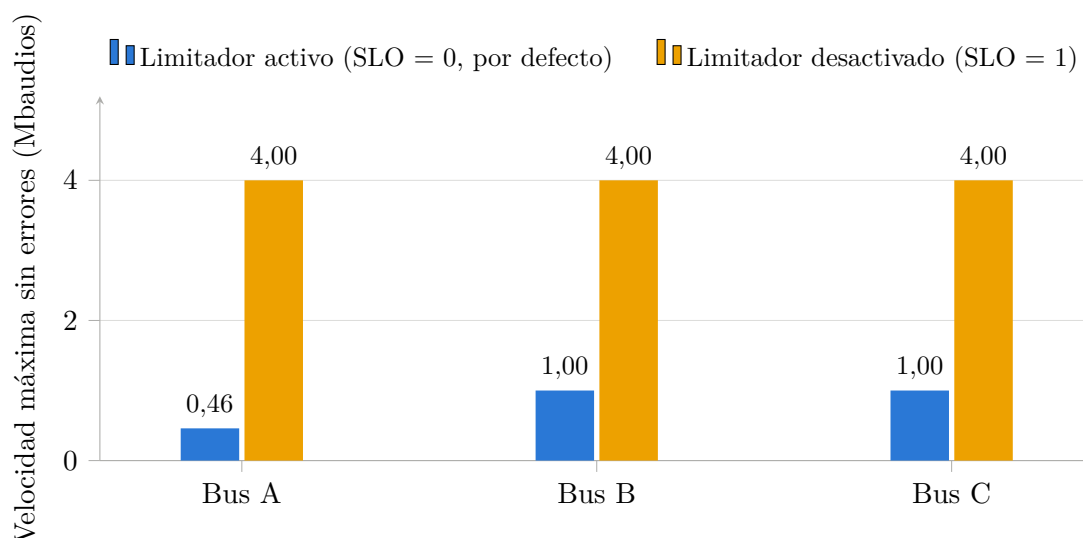
Figura 5.8: Velocidad máxima sin errores en cada bus según el valor del bit SLO.
