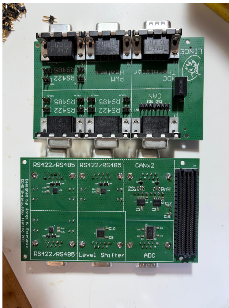
Figura 4.10: Placa CDHS tras el proceso de soldadura.
