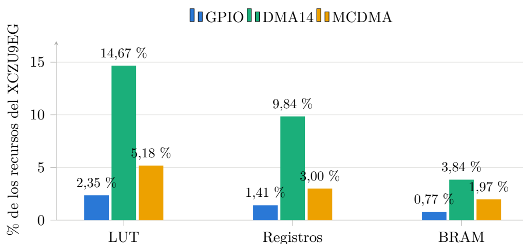
Figura 5.10: Ocupación de la FPGA por variante.
