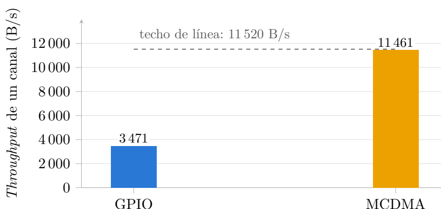
Figura 5.13: Throughput de un canal frente al techo físico de la línea.
