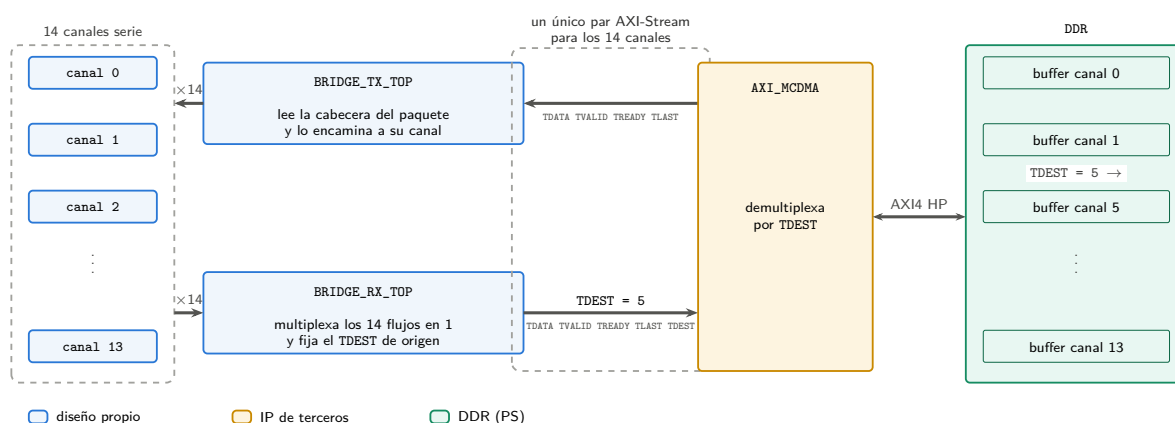
Figura 3.5: Multiplexado de los catorce canales por TDEST.
