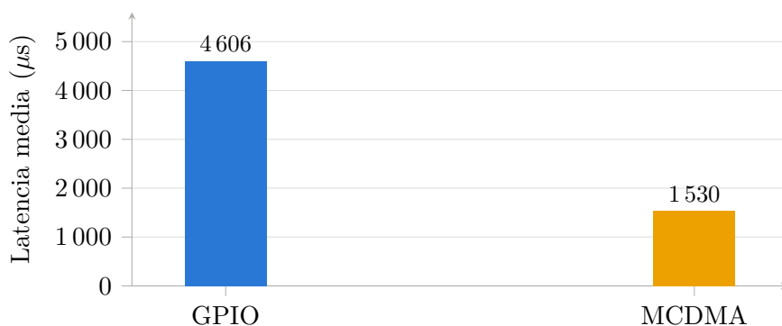
Figura 5.12: Latencia media de entrega de un frame de 11 bytes.
