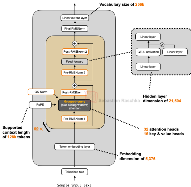
Gemma 3 27B
