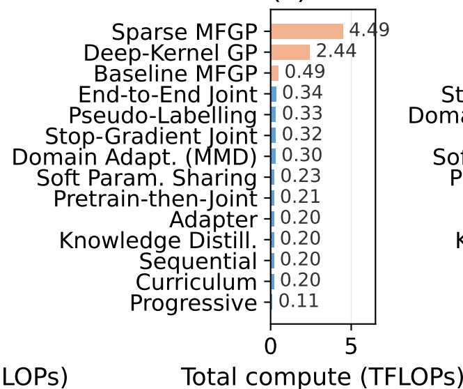
(b) Branin-Unfav
