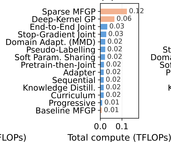
(d) Park-Unfav
