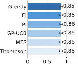
j HOPV15
