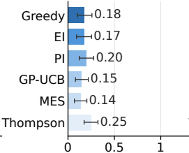
i Polarizability
