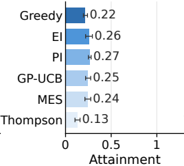
j HOPV15
