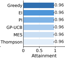
i Polarizability
