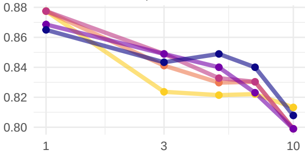
precision
