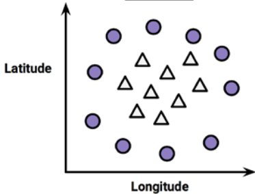
Input Space
