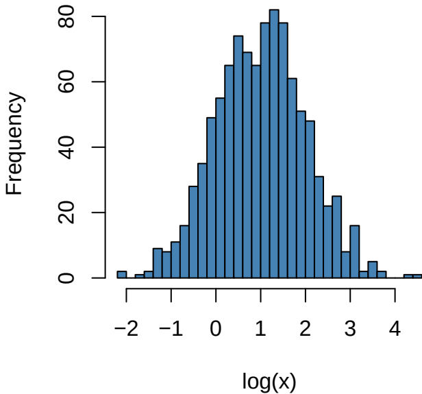
Despues de \log(x)
