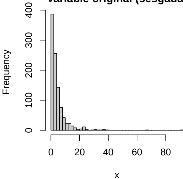
Variable original (sesgada)
