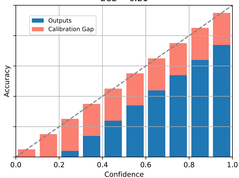
MIMO + Manifold Mixup ECE = 0.21
