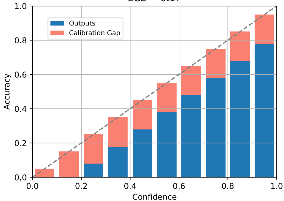
Manifold Mixup ECE = 0.17
