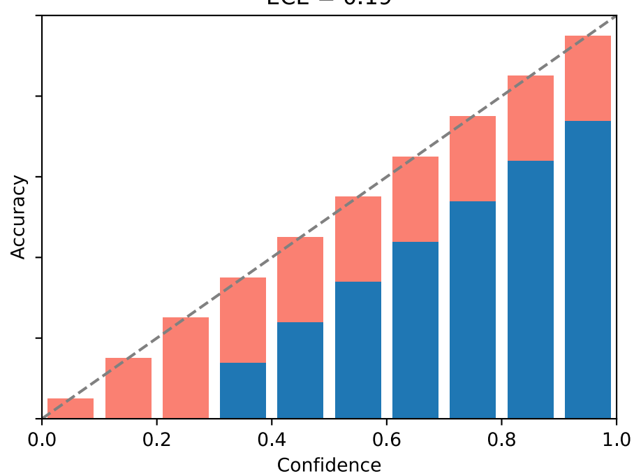
MIMO + Manifold Mixup ECE = 0.19
