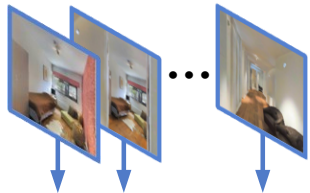
Visual Encoder
