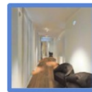
Visual Encoder
