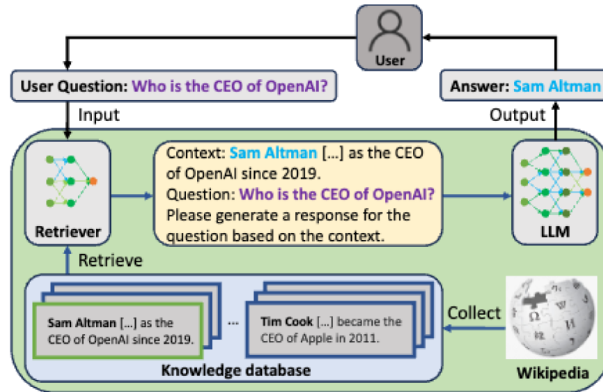
PoisonedRAG; Zou & Geng et al., 2024.
