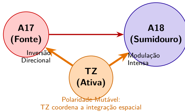
Figure 6 – Mapeamento Evolutivo Topológico do Net-Flow de Informação (Banda Baixa-Gama) . Proporções de entrada ( in-degree ) menos saída ( out-degree ). (A) Durante o período basal, a rede opera numa hierarquia visual preditiva estrita, onde a Área 17 (A17) é o polo motriz primário e a Área 18 (A18) o sumidouro passivo, com a Zona de Transição (TZ) em estado neutro. (B) No exato momento do estímulo (inserção do grating móvel), a topologia sofre uma remodelação ativa. A TZ reverte a sua polaridade passiva e adota dinâmicas de modulação aguda, alterando drasticamente os edge weights (espessura das setas) e provando que a flexibilidade mesoscópica reage transitoriamente à entrada do estímulo periférico.
