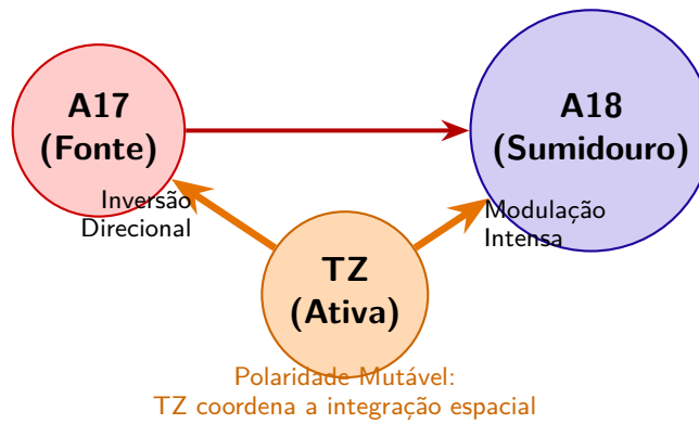
Figure 4 – Mapeamento Evolutivo Topológico do Net-Flow de Informação (Banda Baixa-Gama) . Proporções de entrada ( in-degree ) menos saída ( out-degree ). (A) Durante o período basal, a rede opera numa hierarquia visual preditiva estrita, onde a Área 17 (A17) é o polo motriz primário e a Área 18 (A18) o sumidouro passivo, com a Zona de Transição (TZ) em estado neutro. (B) No exato momento do estímulo (inserção do grating móvel), a topologia sofre uma remodelação ativa. A TZ reverte a sua polaridade passiva e adota dinâmicas de modulação aguda, alterando drasticamente os edge weights (espessura das setas) e provando que a flexibilidade mesoscópica reage transitoriamente à entrada do estímulo periférico.
